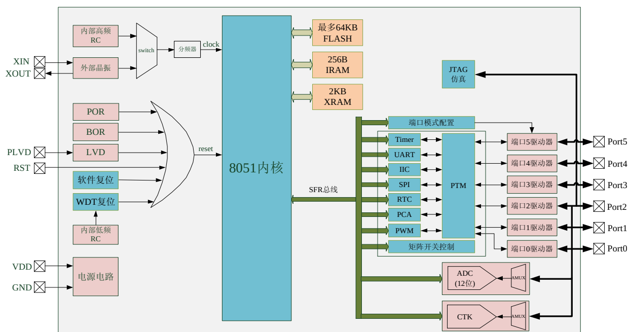
Figure 1-1 系统框图
