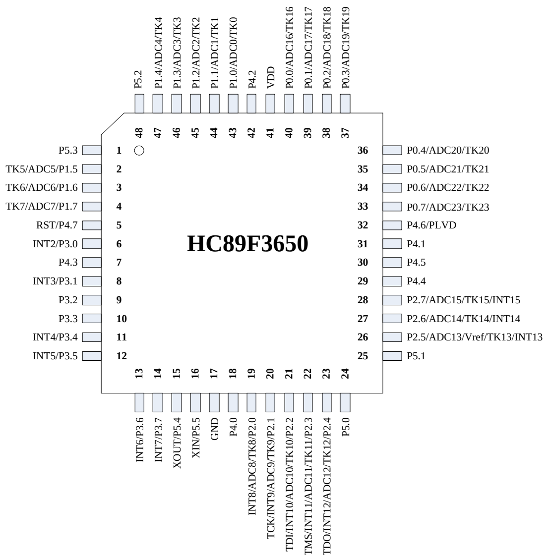
Figure 1-2 LQFP48 引脚配置图
