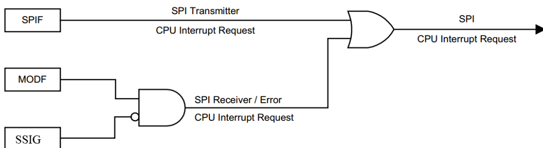
Figure 15-6 SPI 中断请求的产生
