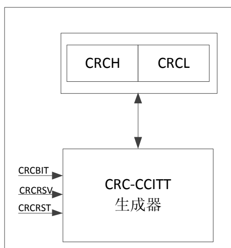
Figure 20-1 CRC 功能框图
