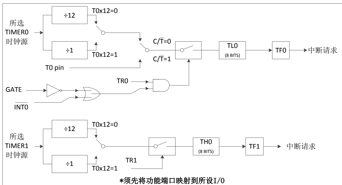
Figure 9-4 TIMER0 方式 3 功能框图
