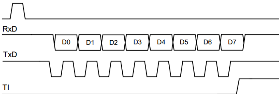
Figure 14-2 模式 0 数据发送时序框图
