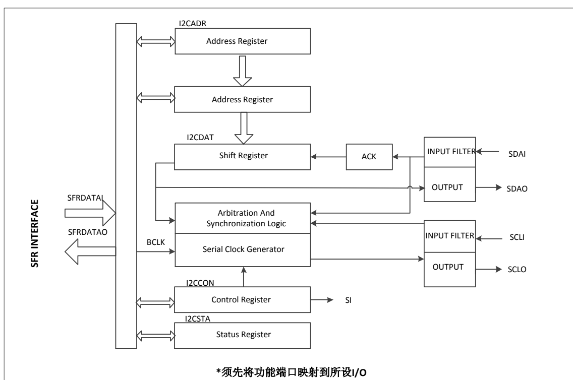
Figure 16-1 IIC 功能框图
