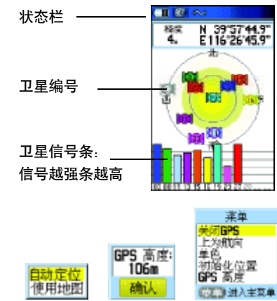
图 2-1 卫星分布图
