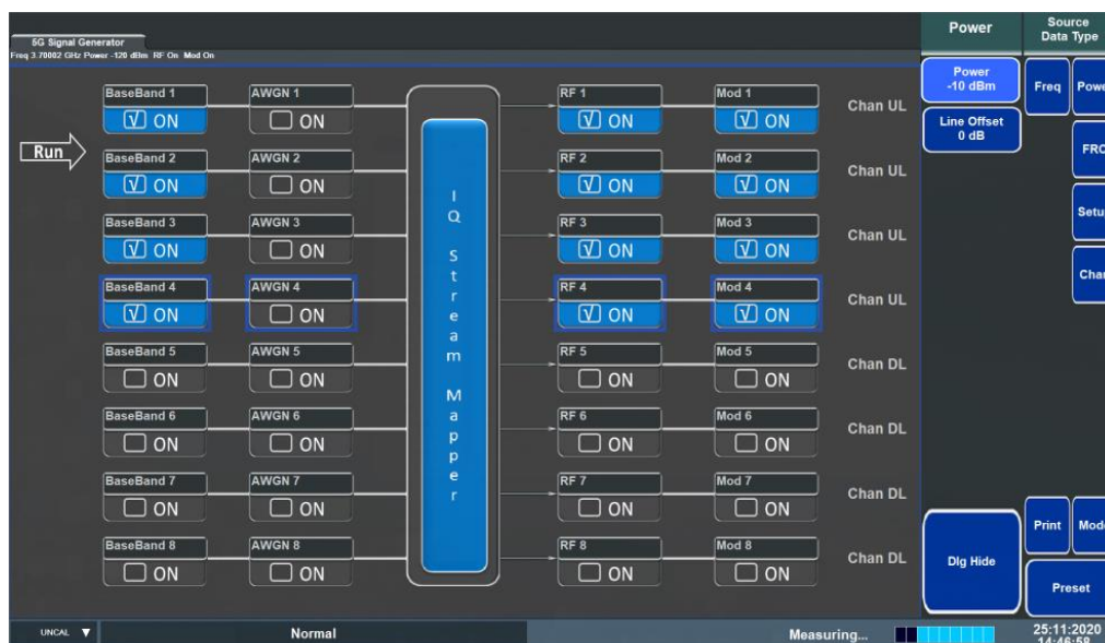
多通道发射
