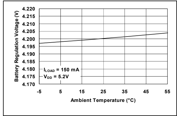
图 2-4: 电池调节电压 ( V_{BAT} ) — 环境温度 ( T_A )
