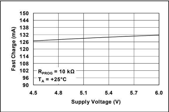
图 2-9: 充电电流 ( I_{OUT} ) — 可编程电阻 ( R_{PROG} )
