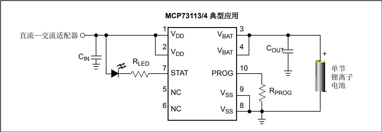
图 6-1: 典型应用电路
