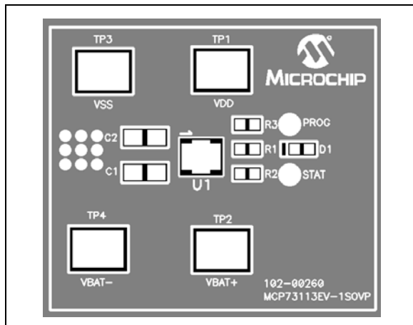
图 6-3: 典型布局 (顶层)
