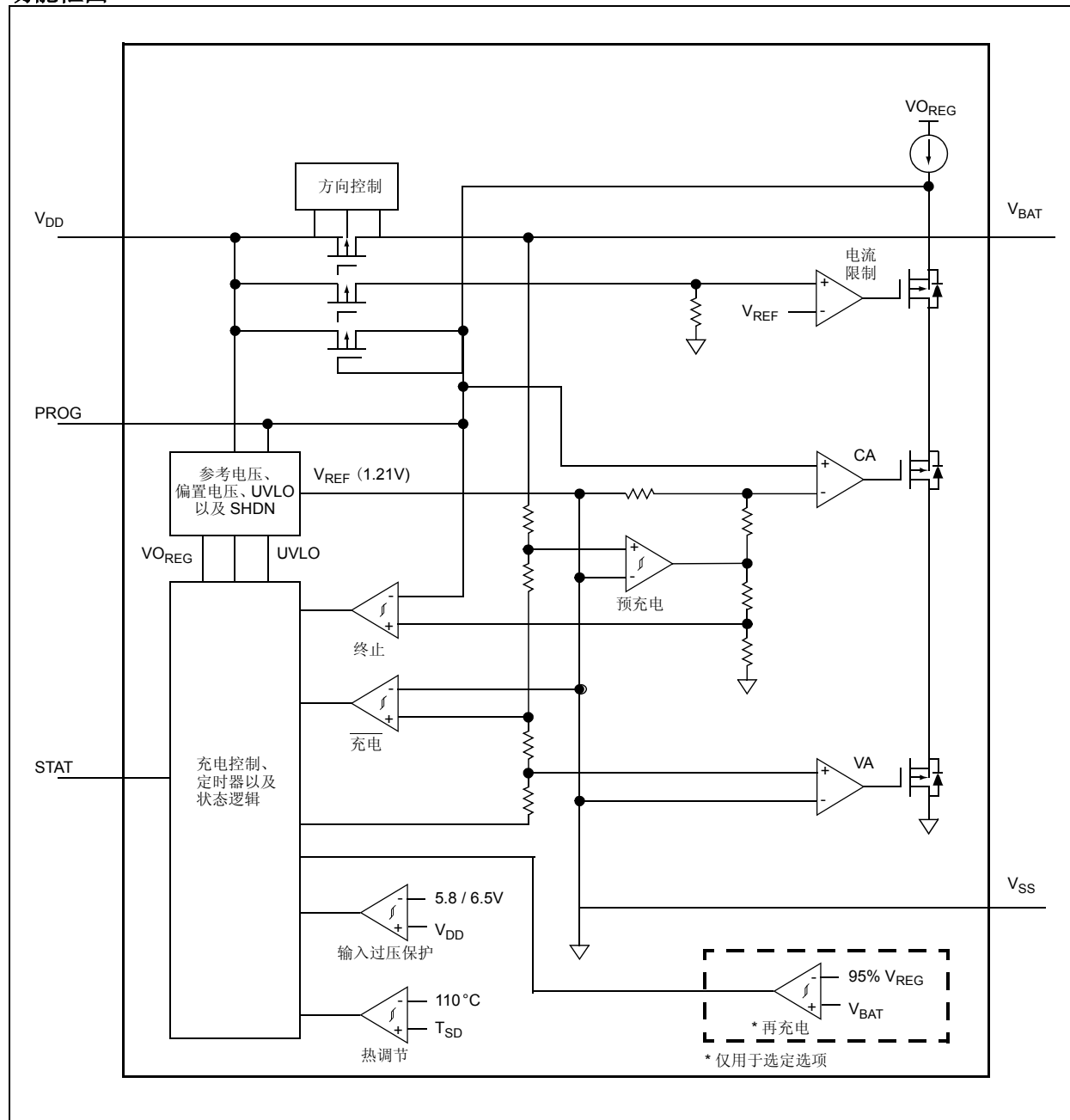
功能框图
