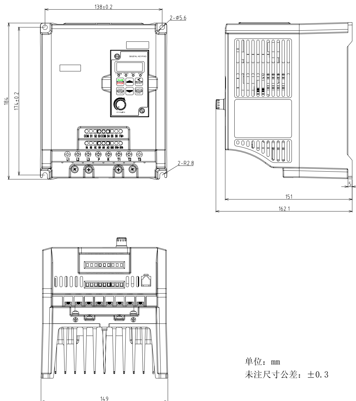
(2) 型 2: 三相: E310-403/405
