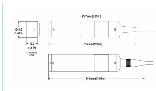
PS1000 外形尺寸
