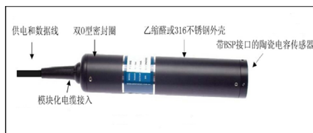
PS1000 结构示意图
