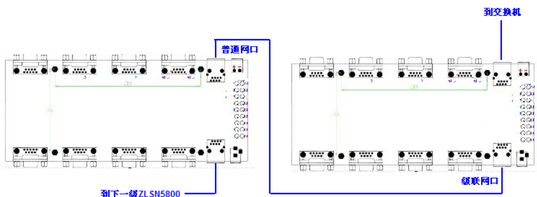
图 5 ZLAN5843A 级联方法
