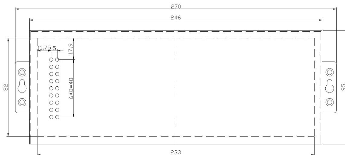
图 6 ZLAN5843A 安装尺寸
