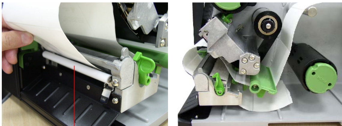
剝紙滾輪
