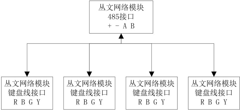
485 总线扩展通信模块结构示意图
