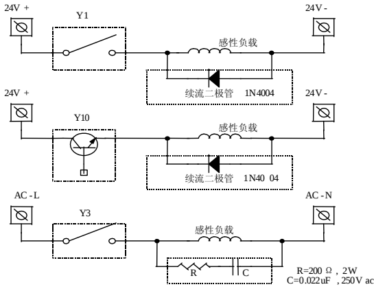
图九 感性负载吸收电路示意图
