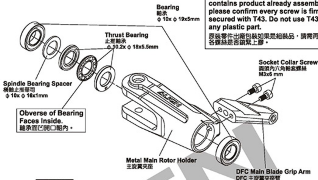
Spindle Bearing Spacer 橫軸止推華司 (φ 10x φ 16x1mm) x 2
