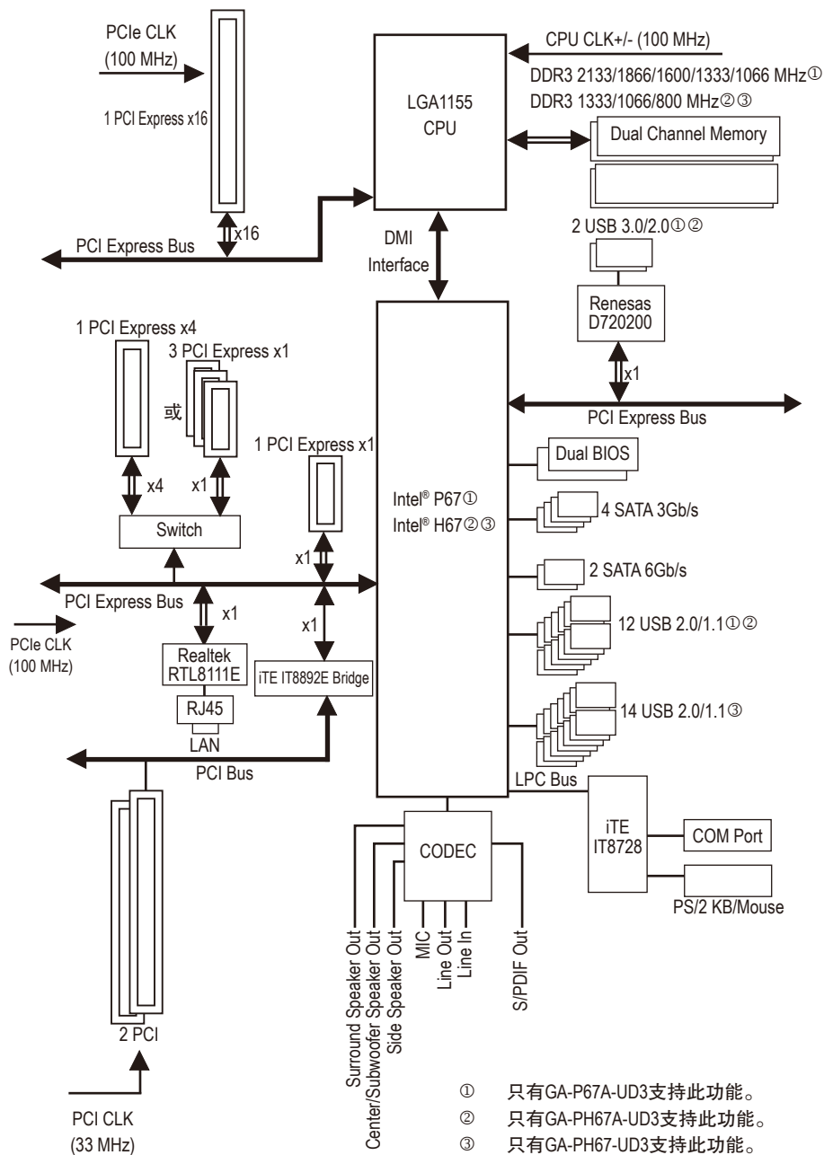
GA-P67A-UD3/GA-PH67A-UD3/GA-PH67-UD3主板功能框图
