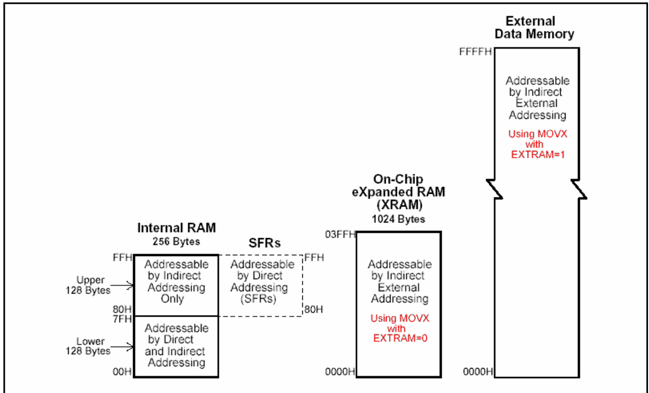
Figure 5-2. 数据存储器
