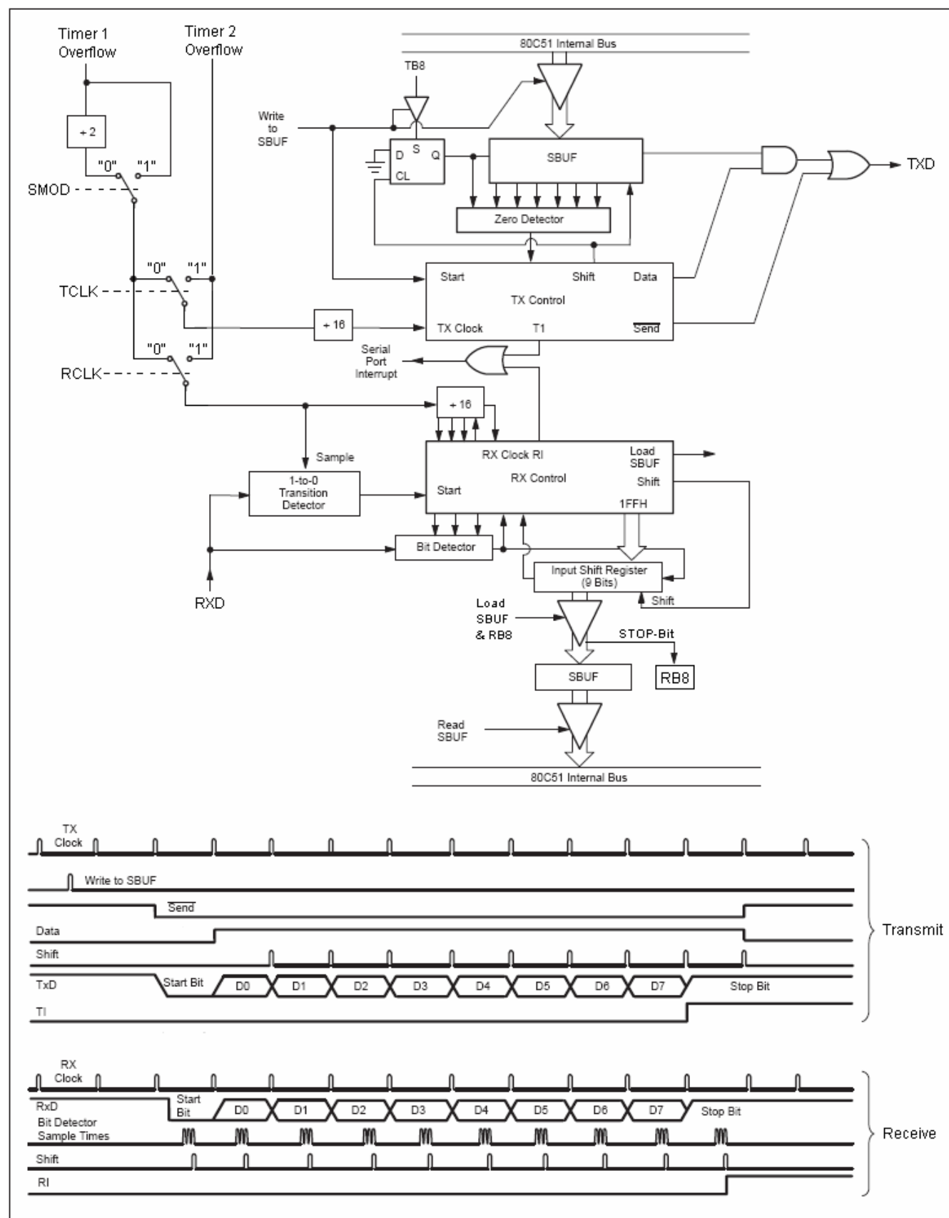
图 12-2 串行口模式 1
