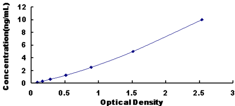
图 1: 人紧密连接蛋白 Claudin 4(CLDN4)试剂盒标准曲线
