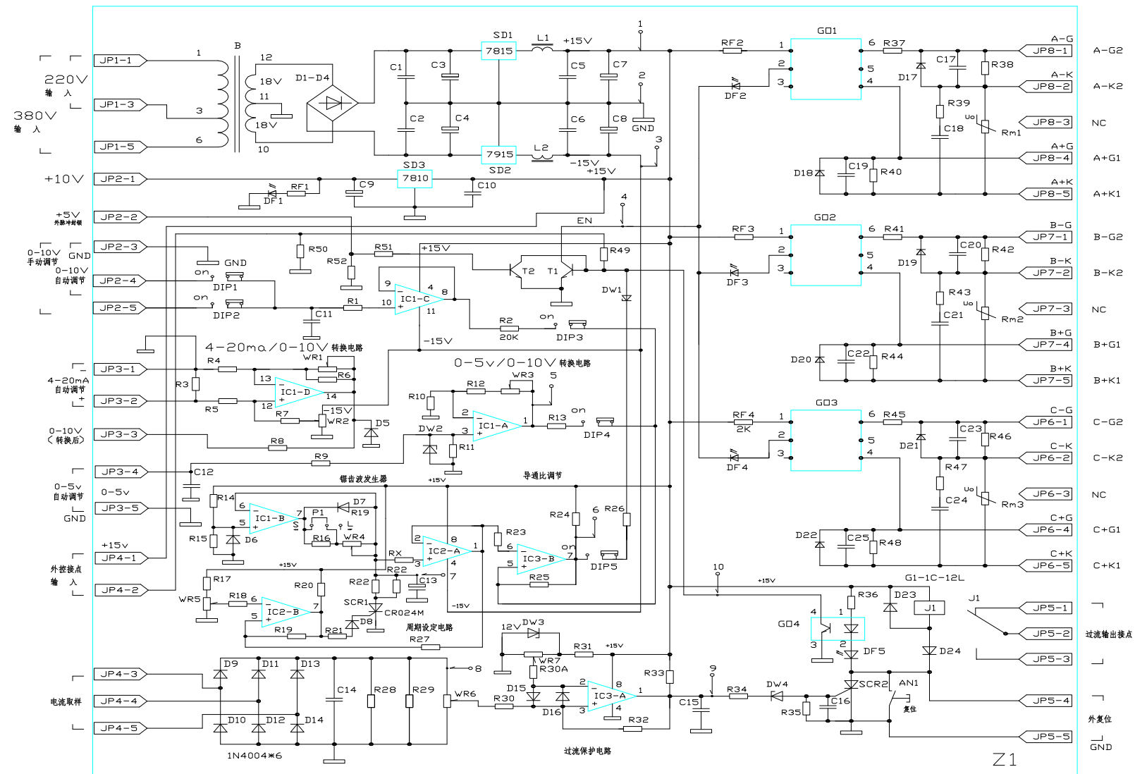
附图一 触发电路板电路原理图
