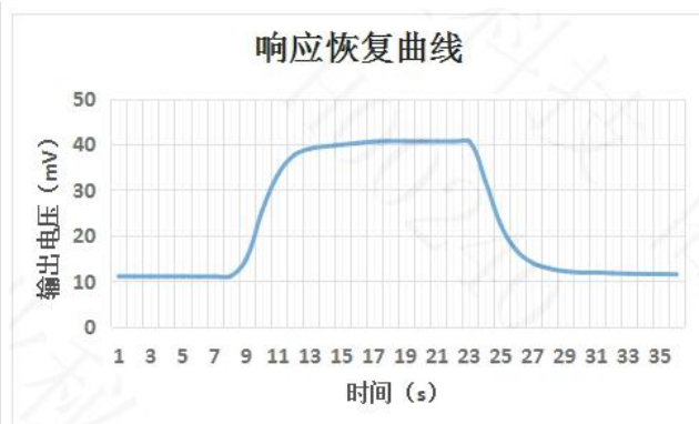
图 4：响应恢复曲线
