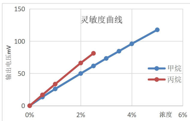
图 3：灵敏度曲线
