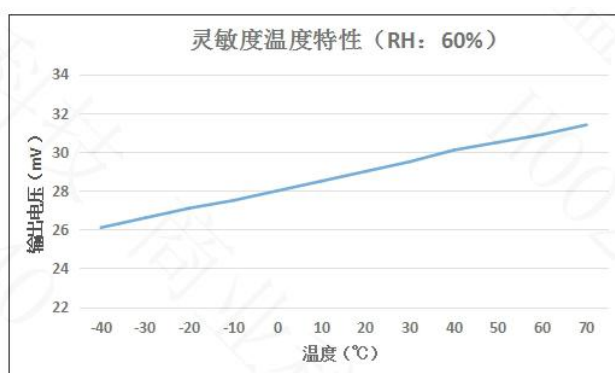
图 6：灵敏度温度特性曲线
