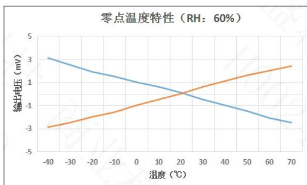
图 5：零点温度特性曲线
