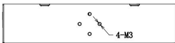
固定片尺寸
