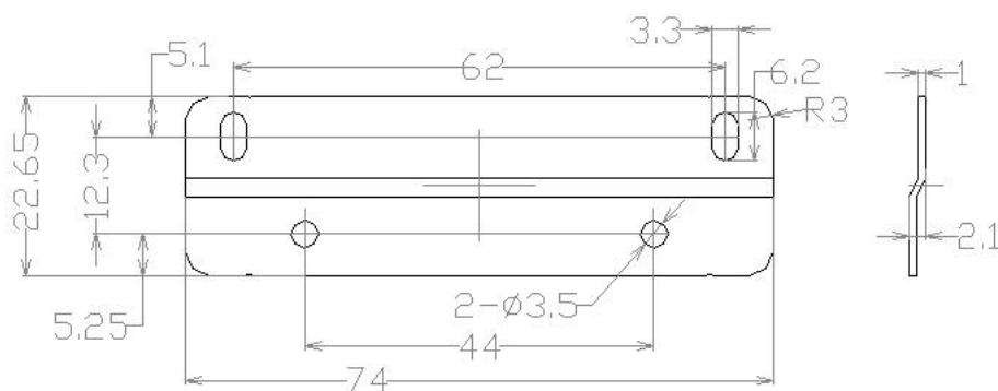
固定片尺寸
