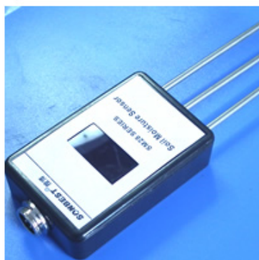
SM2802BD 土壤水分温度传感器 RS485 带液晶显示
