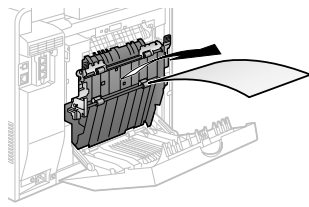
双面组件
