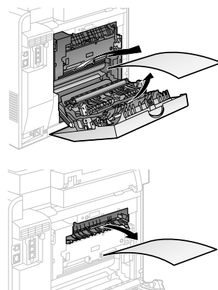
后盖
