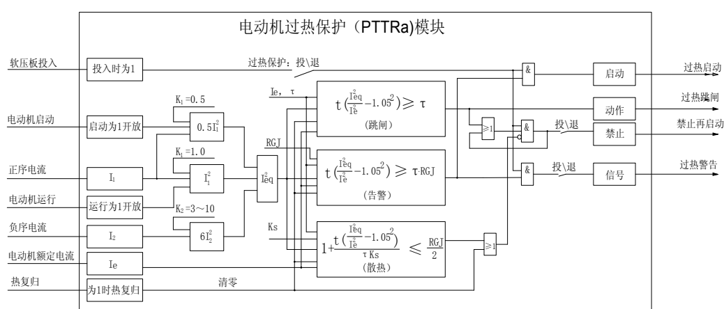
图4-14 电动机过热保护原理框图
