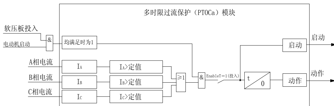
图4-3 启动时间过长保护原理框图
