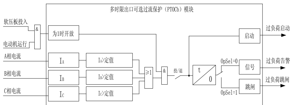
图4-11 过负荷保护原理框图
