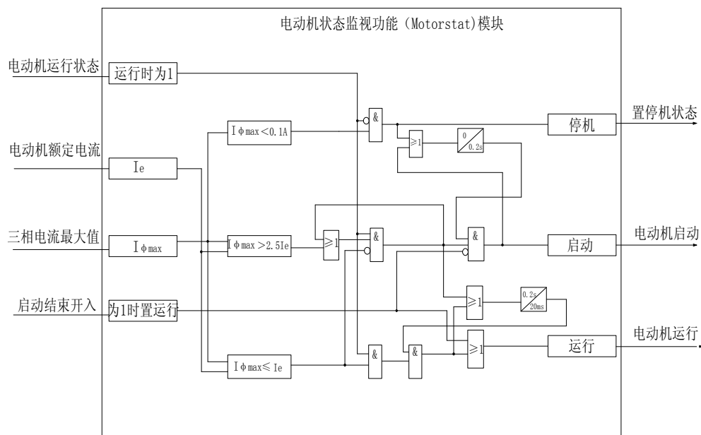
图4-2 电动机状态监视原理框图
