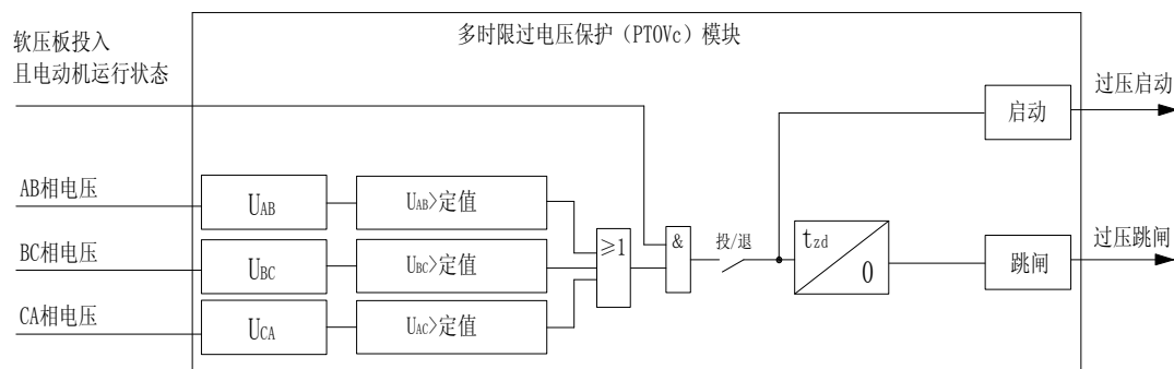
图4-12 过电压保护原理框图
