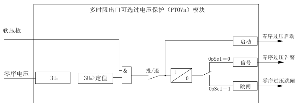
图4-10 零序过压保护原理框图
