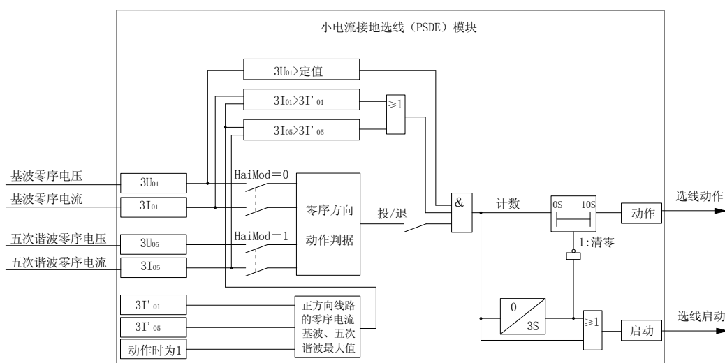
图4-9 小电流接地选线原理框图
