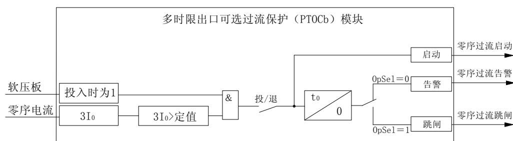
图4-8 零序过流保护原理框图
