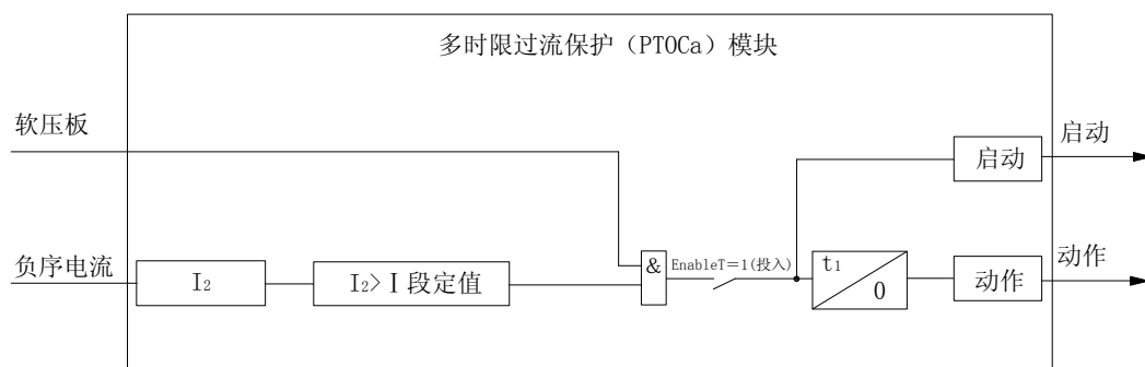
图4-6 负序过流I段保护原理框图
