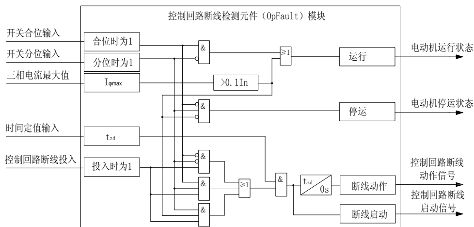
4-17 控制回路断线检测及电动机状态监视原理框图
