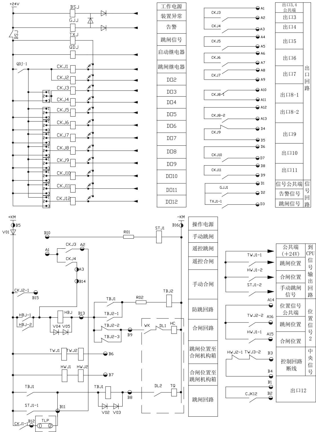
附图 2 DSI 5151 出口及操作回路原理图
