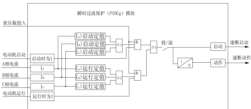
图4-4 速断保护原理框图（过流与速断同）
