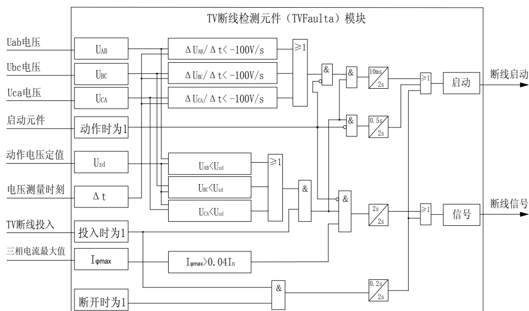
图4-15 TV断线检测元件原理框图
