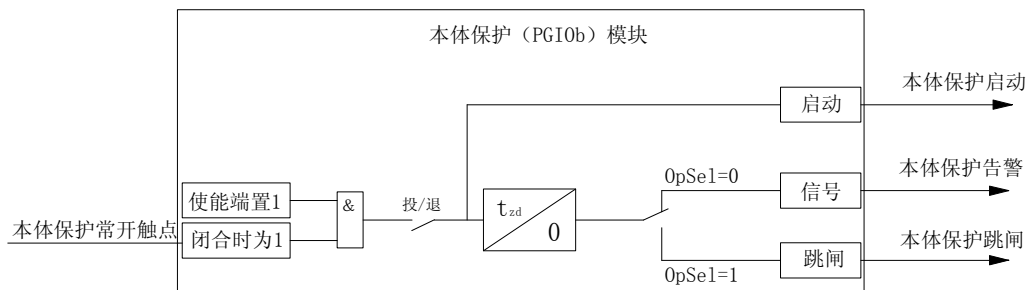
图4-18 本体保护原理框图
