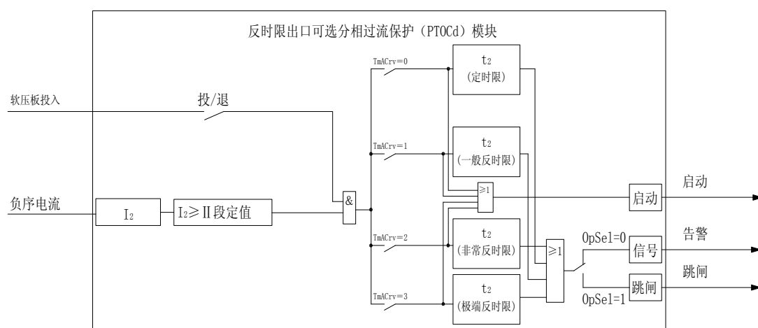
图4-7 负序过流II段保护原理框图
