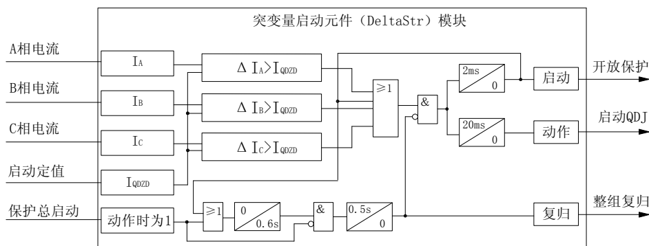
图4-1 启动元件逻辑框图
