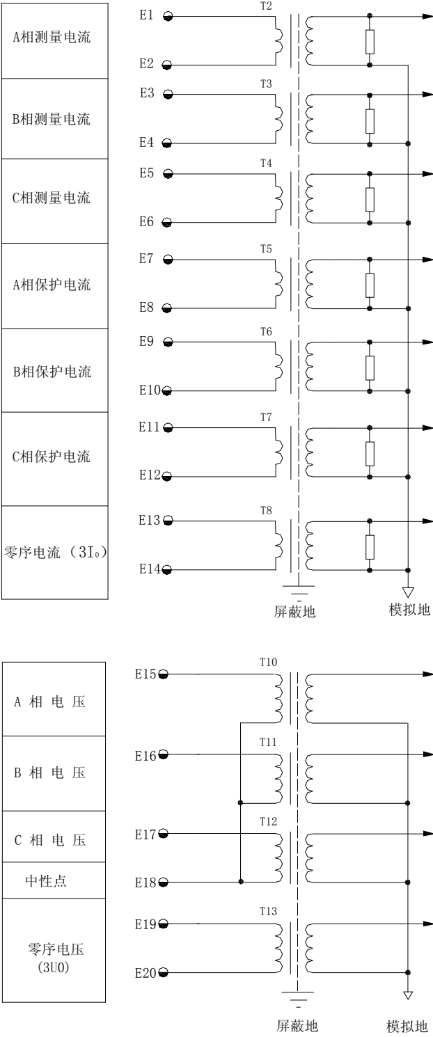
附图1 DSI 5151交流回路原理图
