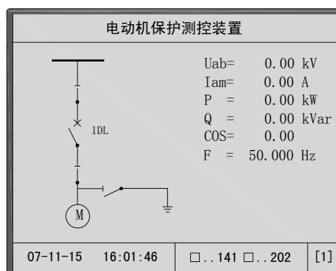
图5—2 静态工作界面
