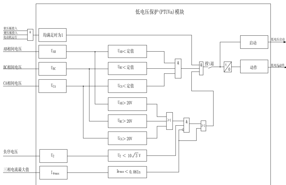
图4-13 低电压保护原理框图
