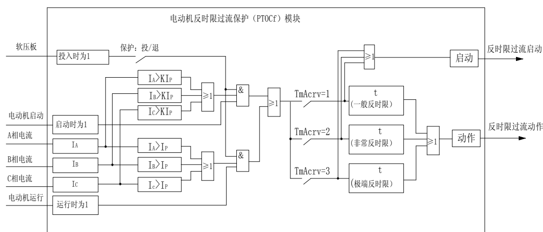
图4-5 反时限过流保护原理框图
