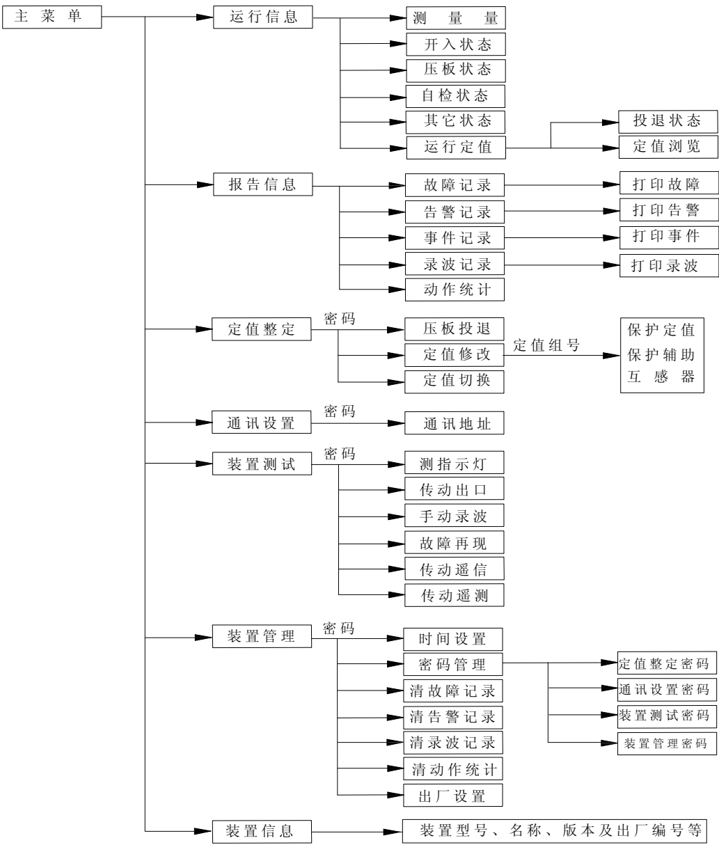
图5-4 液晶界面拓扑图
