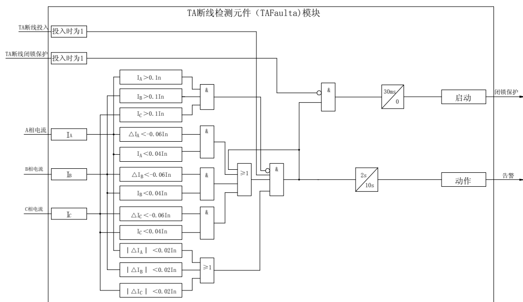
图4-16 TA断线检测元件原理框图
