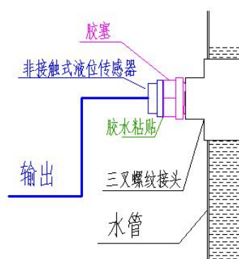
图 5 感应器安装在三叉接头的铁水管（金属、吸水性容器安装示意图）
