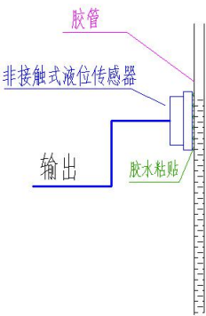
图 6 感应器直贴在胶水管上（绝缘性容器安装示意图）
