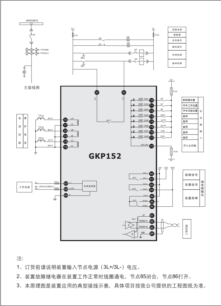
线路保护接线原理图
