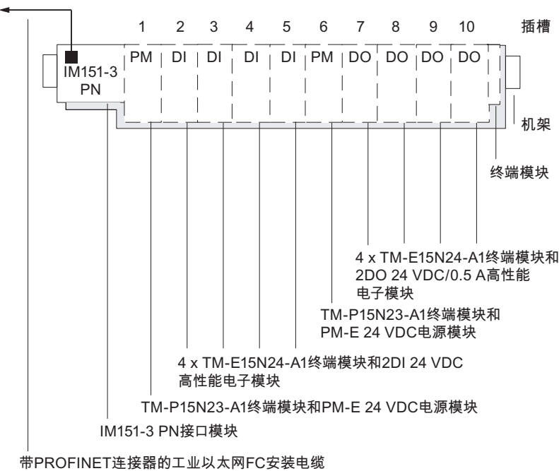
图 2-1 PROFINET IO 上的实例的组件
