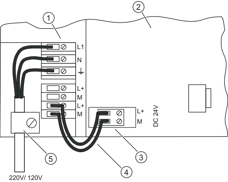
图 3-1 为电源和 CPU 接线（前面板盖打开）
