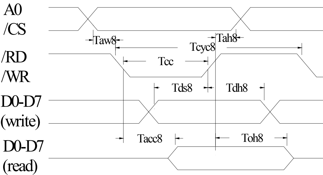
Intel8080 时序表：
