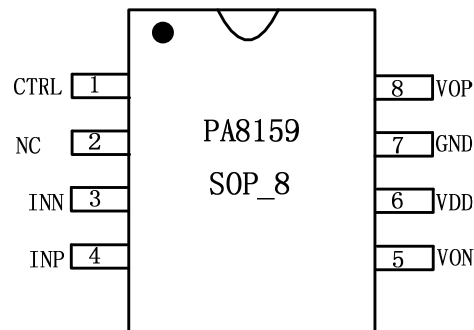
图2. PA8159 封装图
