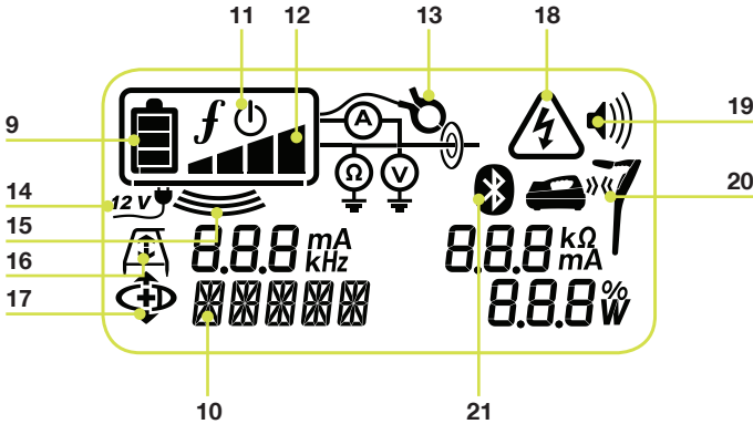
图 2.8: 发射机 LCD
