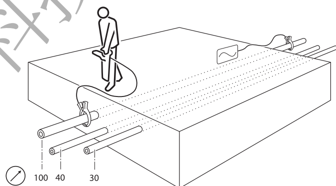
图 10.1: 连接夹钳
