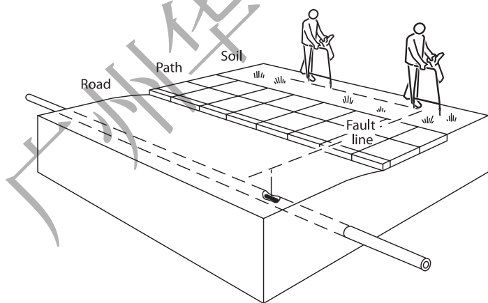
图 11.2: 用接收机和A字架定位故障
