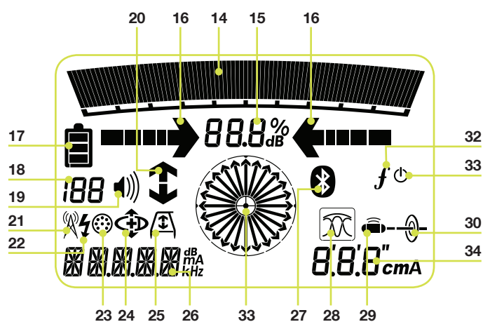
图 2.4: 接收机 LCD
