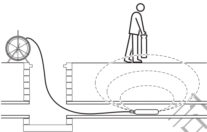
图 10.6: 使用探头
