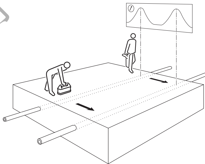
图 7.5: 感应法搜索
