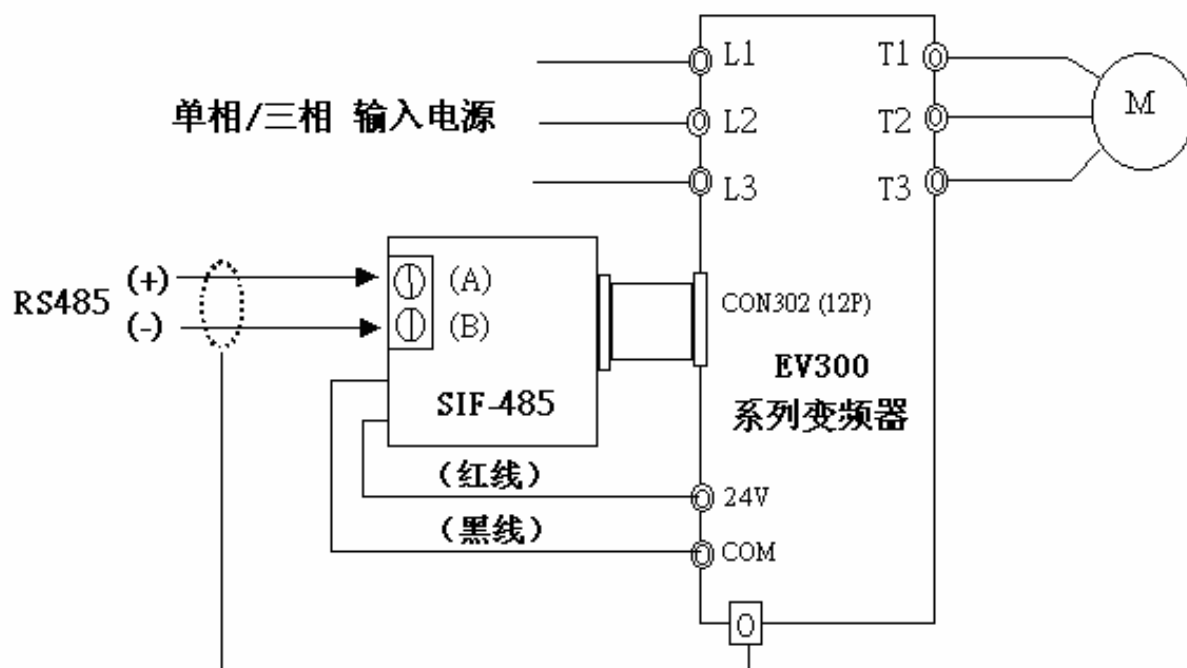
SIF-485 配线图：
