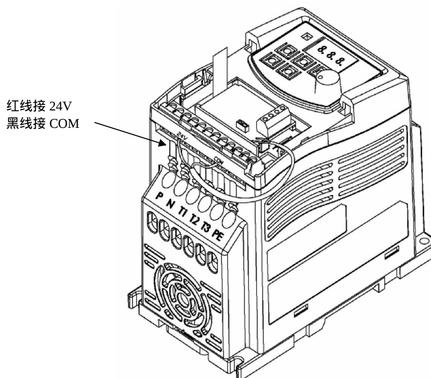
SIF-IO 配线图
