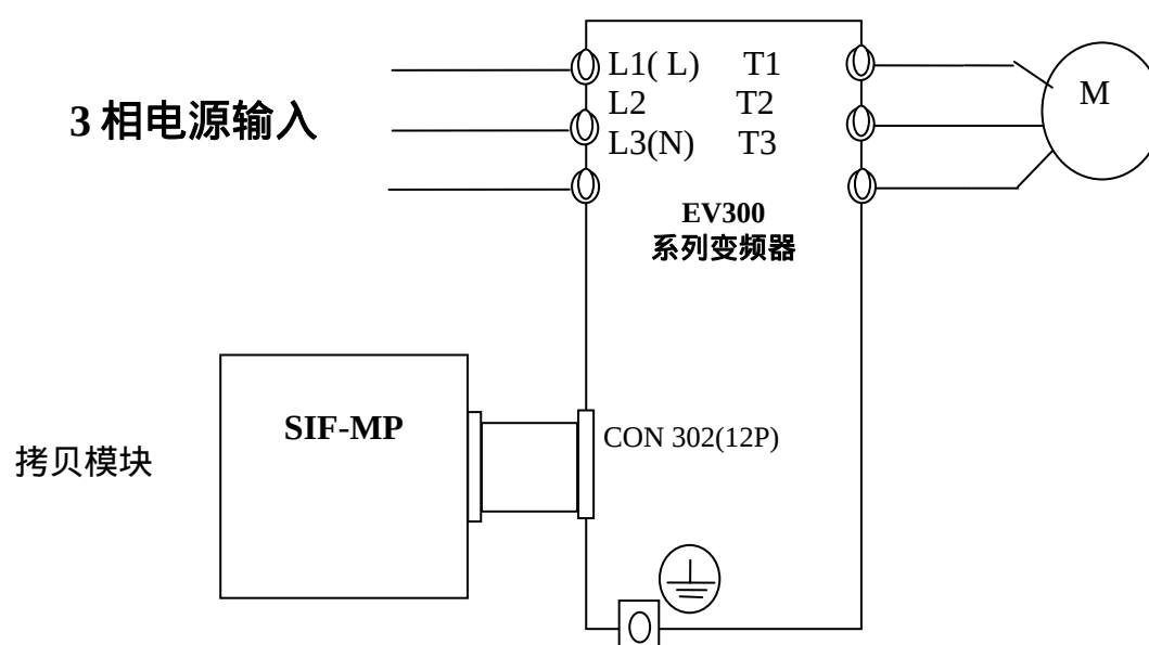
SIF-MP 配线图
