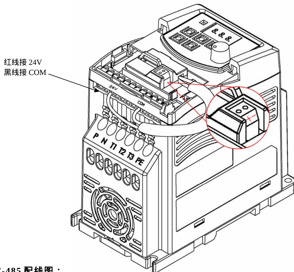
SIF-485 配线图：
