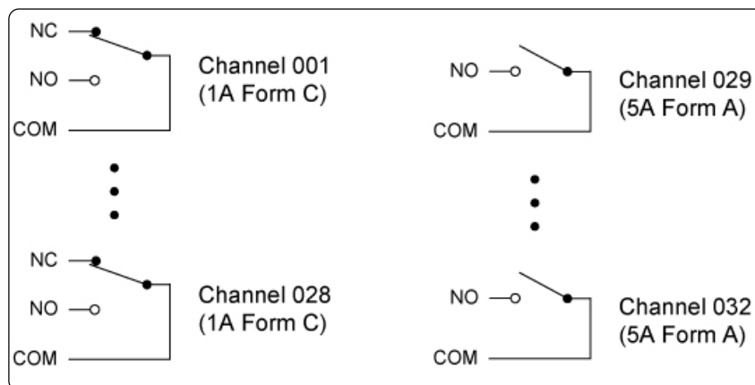
图 1. L4437A 32 通道通用开关
