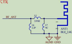
WT8002+WT2605典型应用电路原理图
