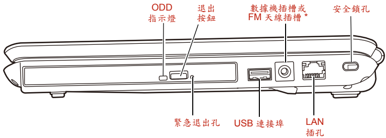
電腦右側圖
