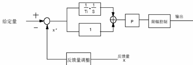
图 5-10 PI 调节原理框图
