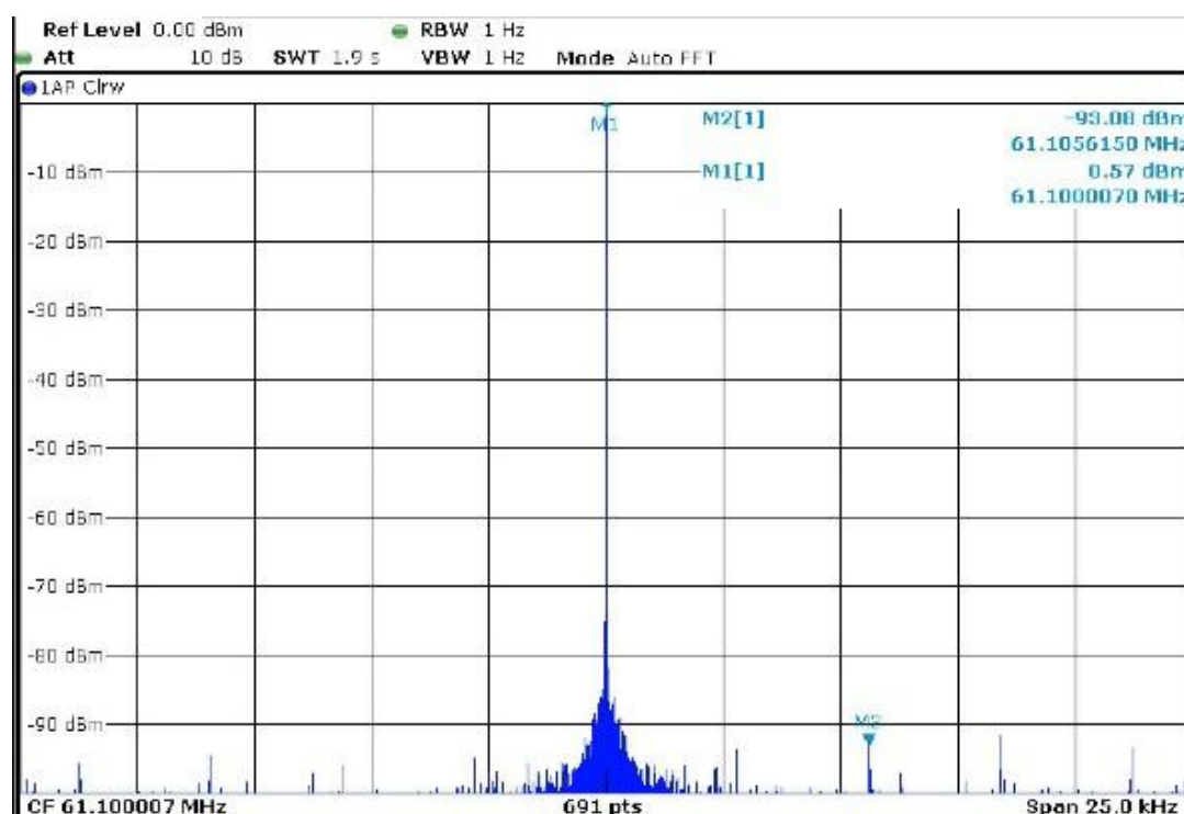
图 6 图 3 的窄带视图 (带有载波和下边带抑制)
