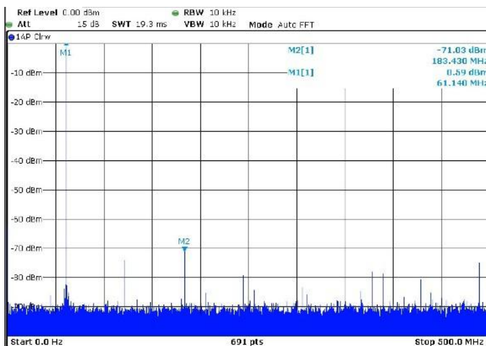
图 3 61.1MHz 条件下的宽带 SFDR, REFCLK=1GHz
