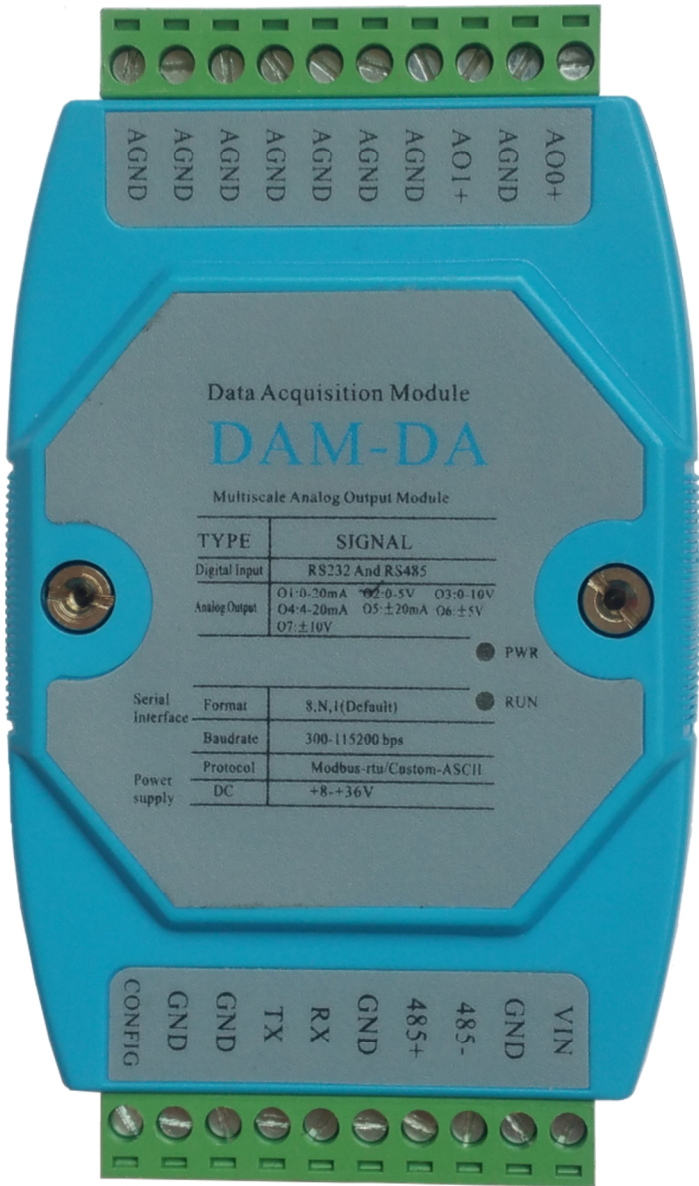
图 1-1 DAM-DA 实物图
