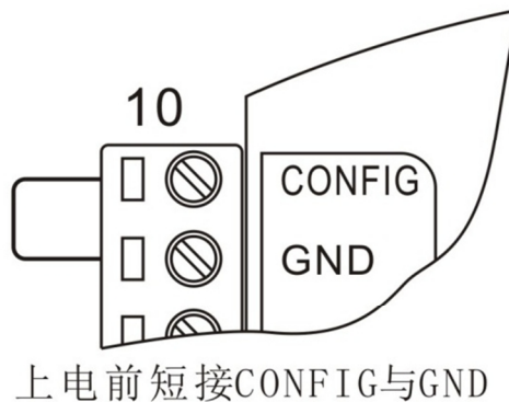
图 6-1 配置模式端口短接示意图
