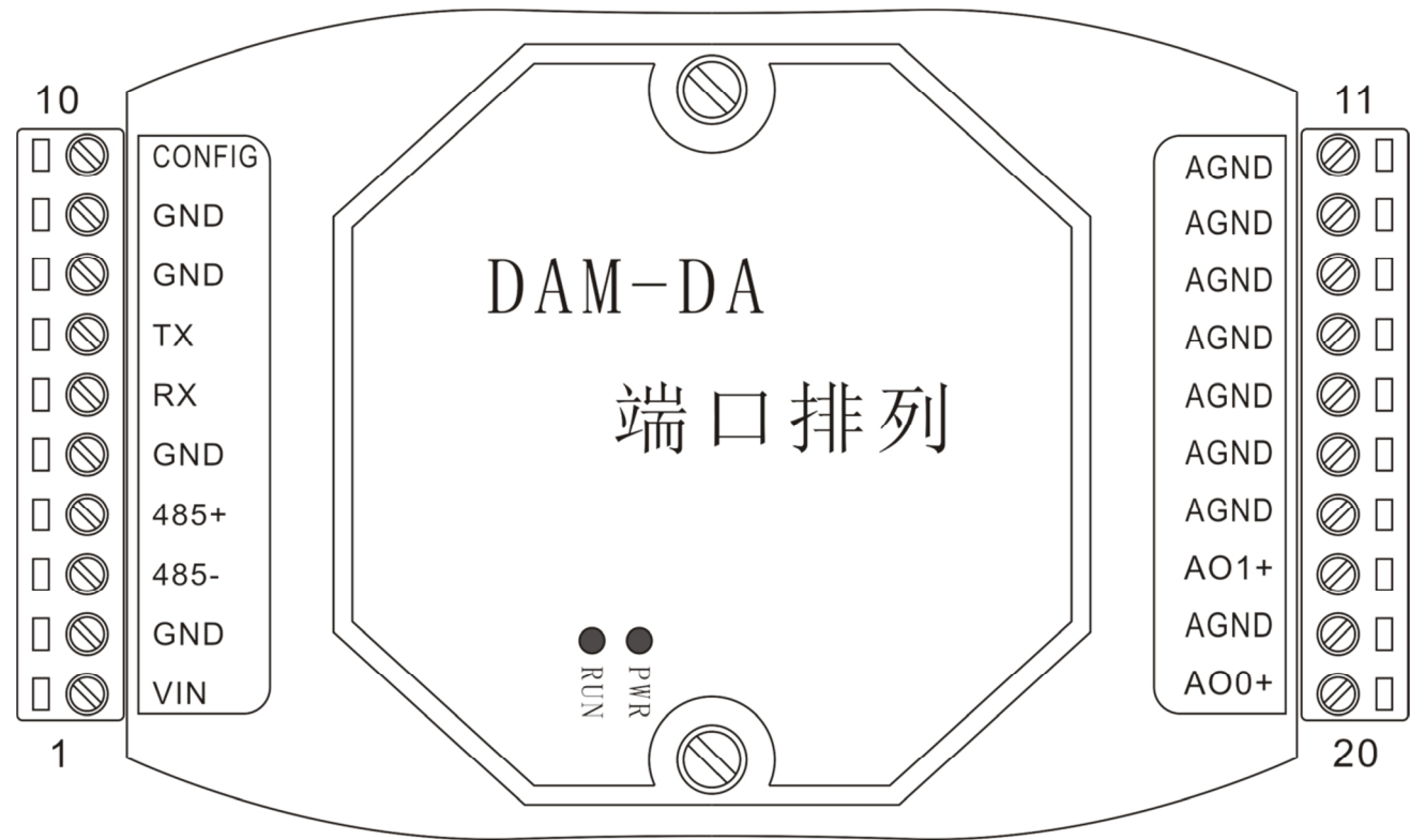
图 4-1 DAM-DA 模块端口位置示意图
