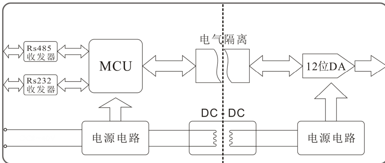
图 1-2 DAM-DA 工作原理框图
