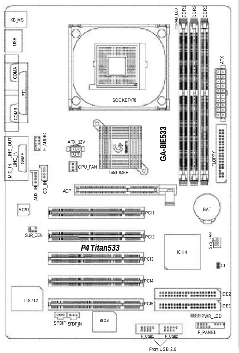
GA-8IE533 主機板 Layout 圖
