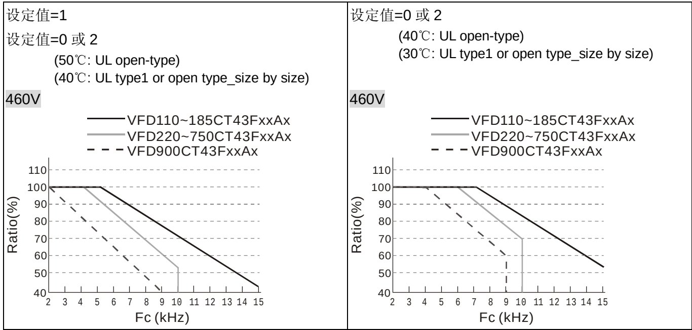
Heavy Duty 之降载曲线图
