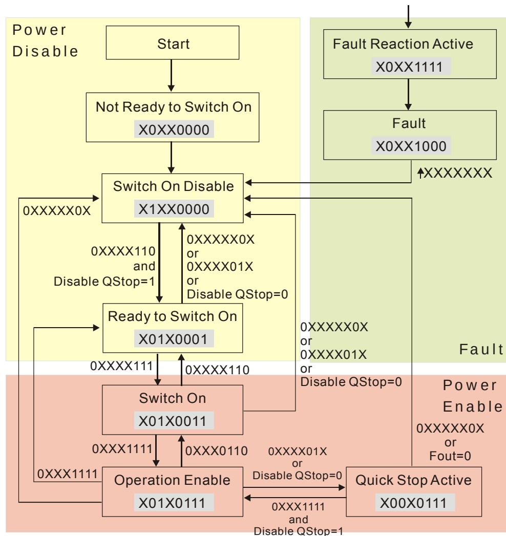
<状态切换流程图>
