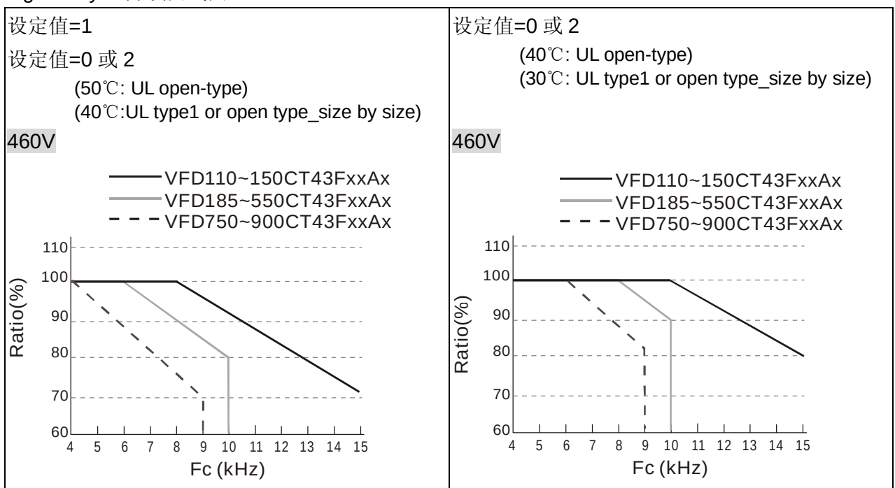
Light Duty 之降载曲线图
