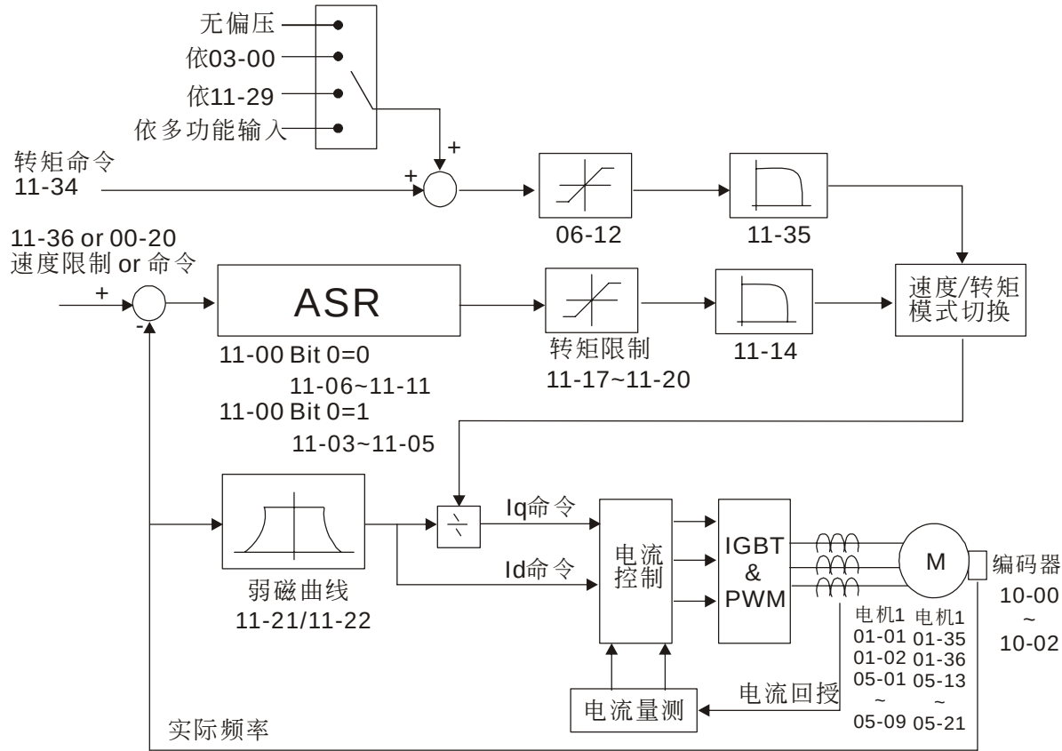
TQCPG 控制方块图如下
