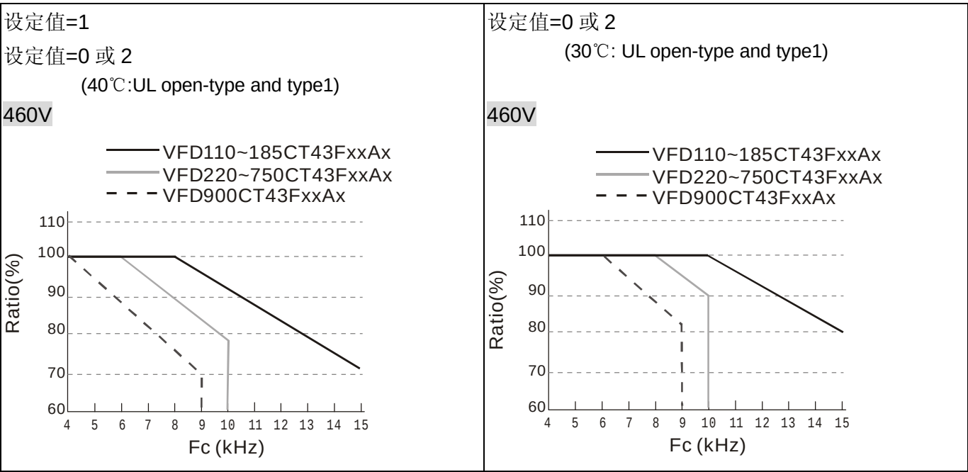
Light Duty 之降载曲线图
