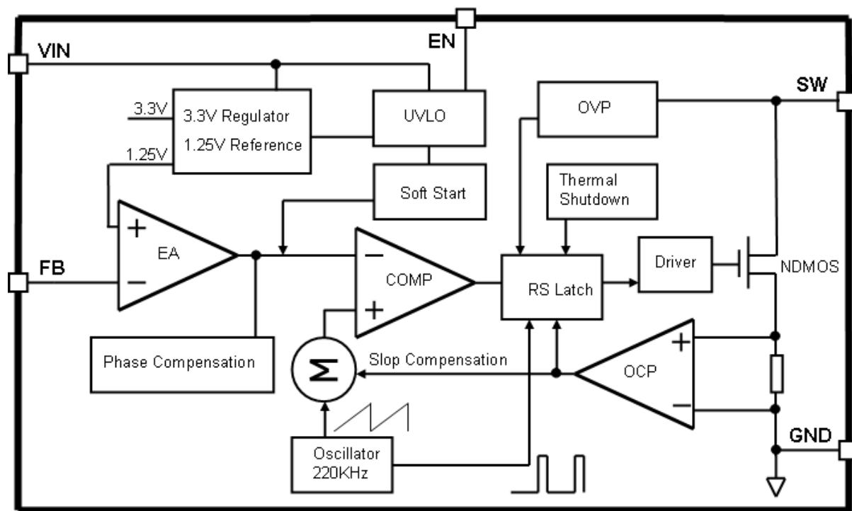
图 3. XL6019 方框图
