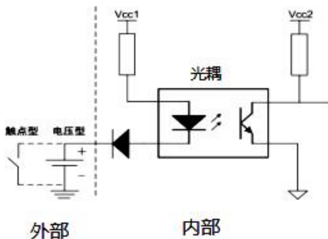
数字量输入原理示意图
