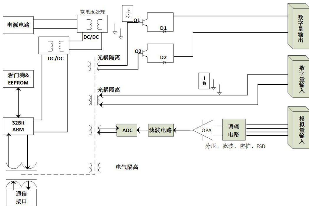
原理框图
