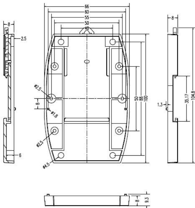
亚当盒机械尺寸示意图
