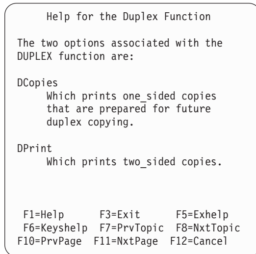
Figure 152. Parameter terms
