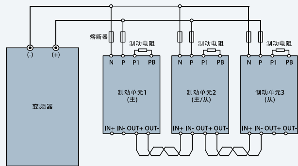
制动单元并联接线方式 1
