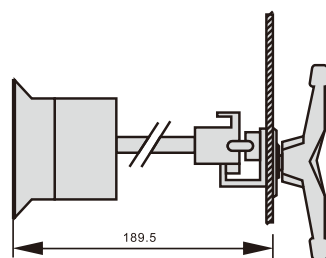
RDH5Z2-800A~ 1600A柜外操作
