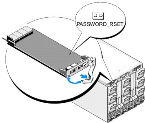
Ilustración 11-1. Ubicación del puente de restablecimiento de contraseña
