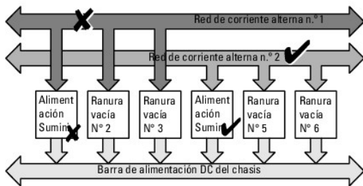
Ilustración 8-2. Nivel de redundancia 2+2
