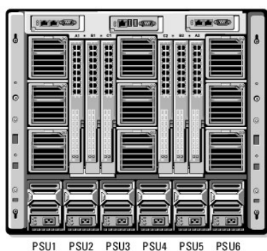
Ilustración 8-6. Chasis con configuración de seis unidades de suministro de energía
