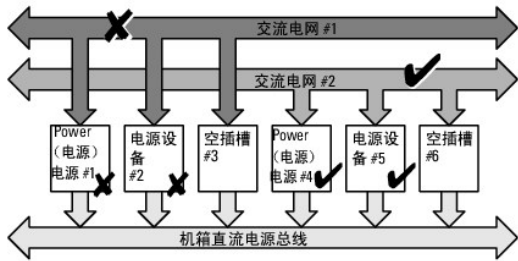
1 3+3 交流冗余级别 — 每个电网连接三个 PSU。因为三个 PSU 可为整个机壳加电，所以此配置不受一个交流电网整体故障的影响，不会损失为机壳提供的电源。
