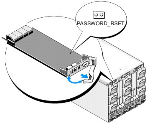
图 11-1. 密码重设跳线位置
