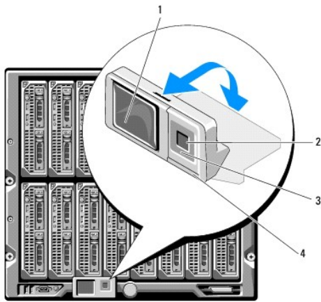
图 2-2. LCD 显示屏
