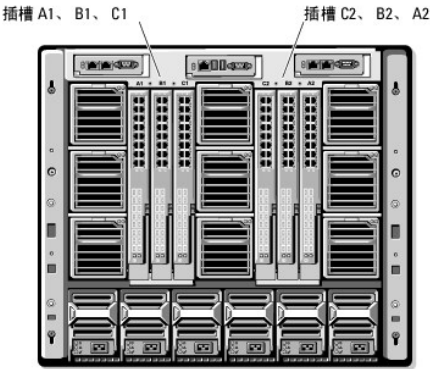
图 10-1. 机箱后视图，显示 IOM 的位置
