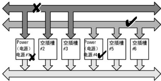
1 2+2 交流冗余级别 — 每个交流电网至少连接两个 PSU。
