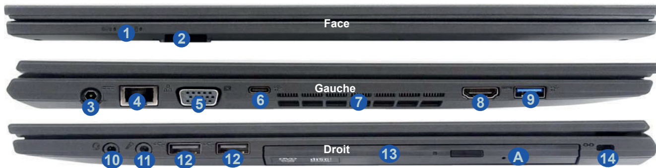
Figure 5 - Vues de face, gauche et droite (Modèle B)
