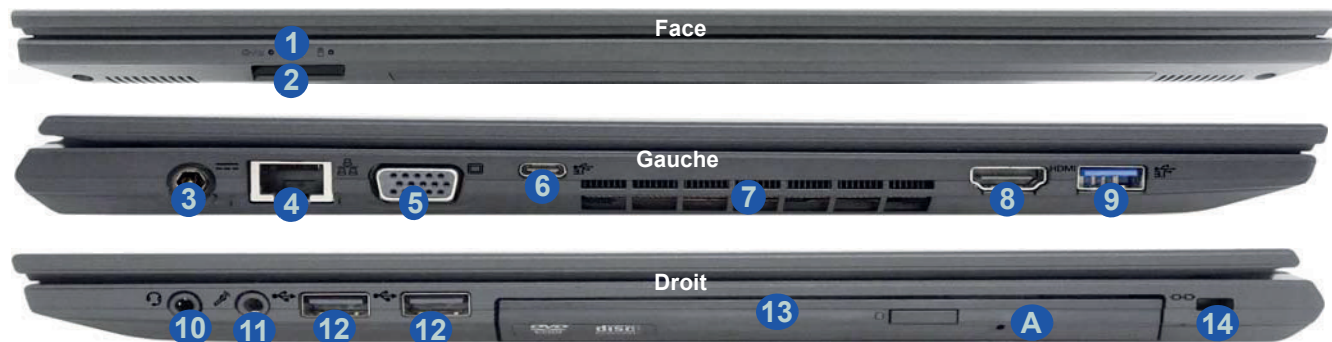
Figure 4 - Vues de face, gauche et droite (Modèle A)
