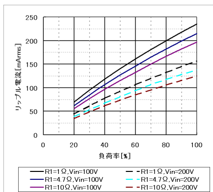
(C) TUHS10(参考値) Cbc=47uF、120Hz時
