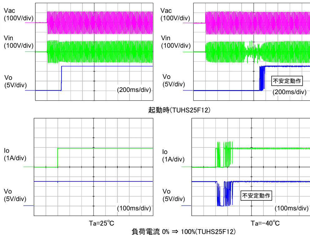
図4.1 温度による 動作の差異
