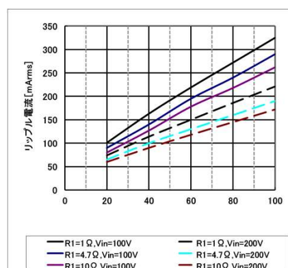
(D) TUHS15(参考値) Cbc=68uF、120Hz時
