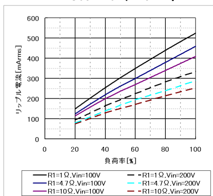
(E) TUHS25(参考値) Cbc=120uF、120Hz時
