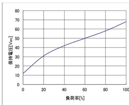
(D)TUHS15 保持電圧(参考値)
