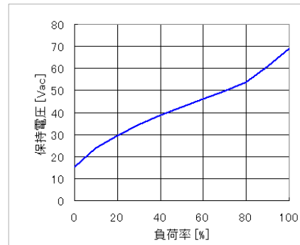
(B)TUHS5 保持電圧(参考値)
