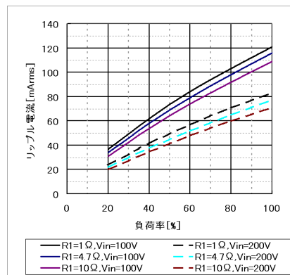
(B) TUHS5(参考値) Cbc=22uF、120Hz時
