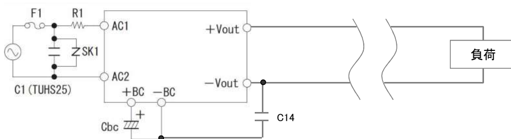
図6.4 1次-2次コンデンサ 接続図
