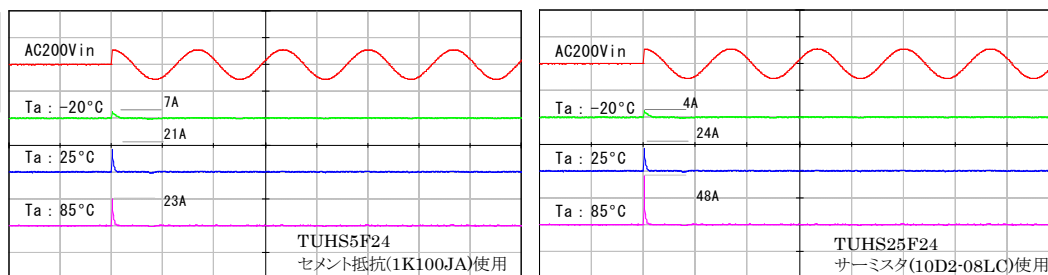
図2.5 突入電流値
