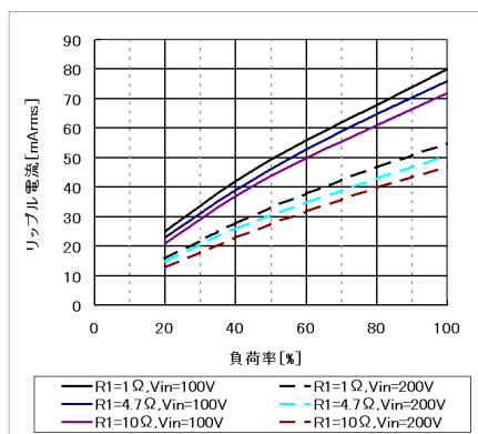
(A) TUHS3(参考値) Cbc=18uF、120Hz時
