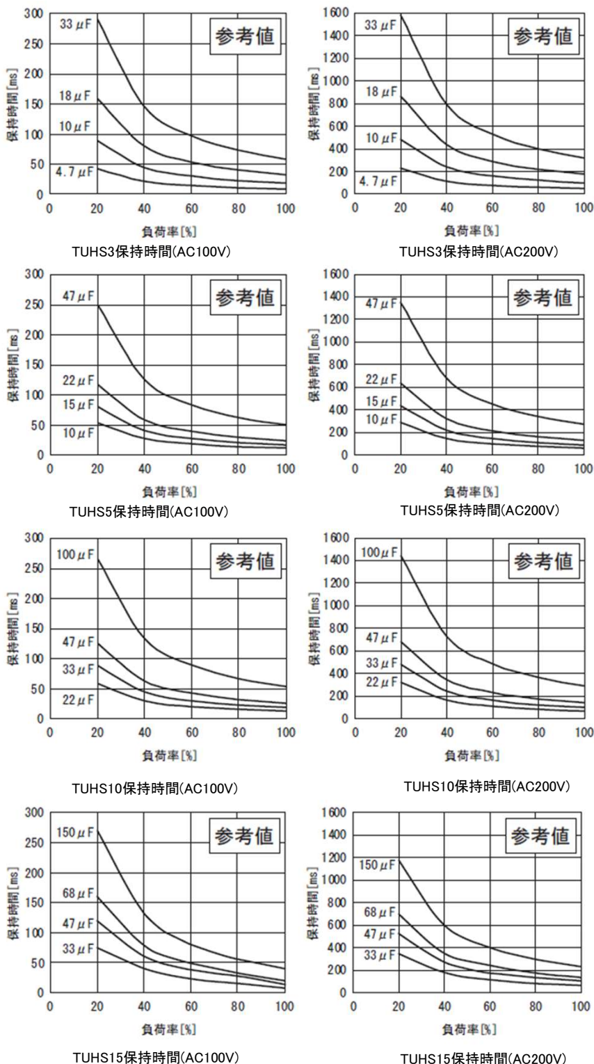
図5.1 保持時間と Cbc容量値との 関係性
