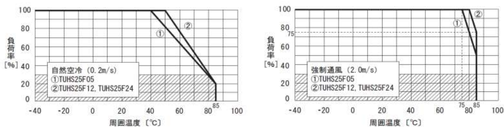
(E) TUHS25(参考値)
