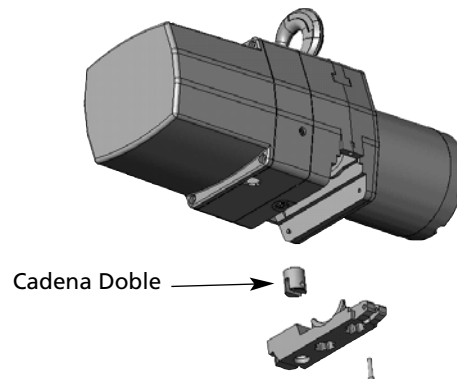
Figura 4 — Diagrama para cambiar la cadena
