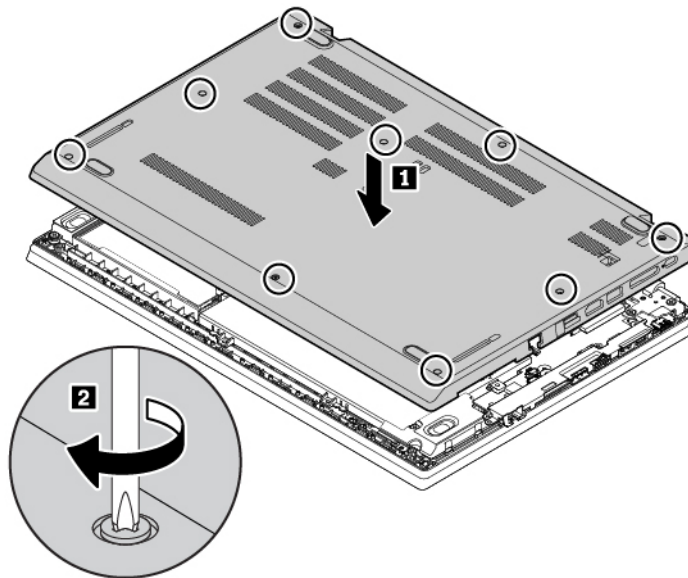
Figure 7. Installation du cache de la base pour les ordinateurs ThinkPad L580
