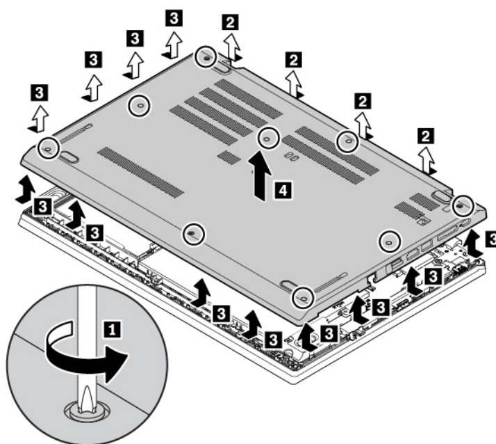
Figure 5. Retrait du cache de la base pour les ordinateurs ThinkPad L580
