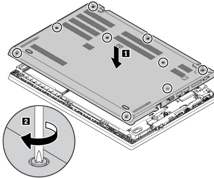
Figure 6. Installation du cache de la base pour les ordinateurs ThinkPad L480
