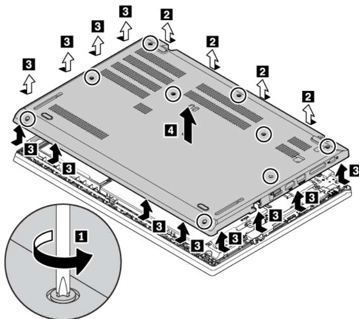
Figure 4. Retrait du cache de la base pour les ordinateurs ThinkPad L480
