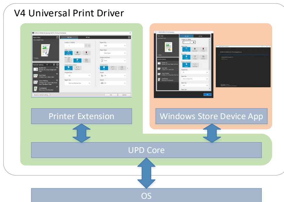
図 2.2-1 V4 UPD の構成
