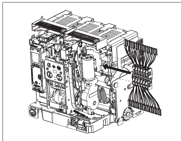
图32. 右侧附件盘
