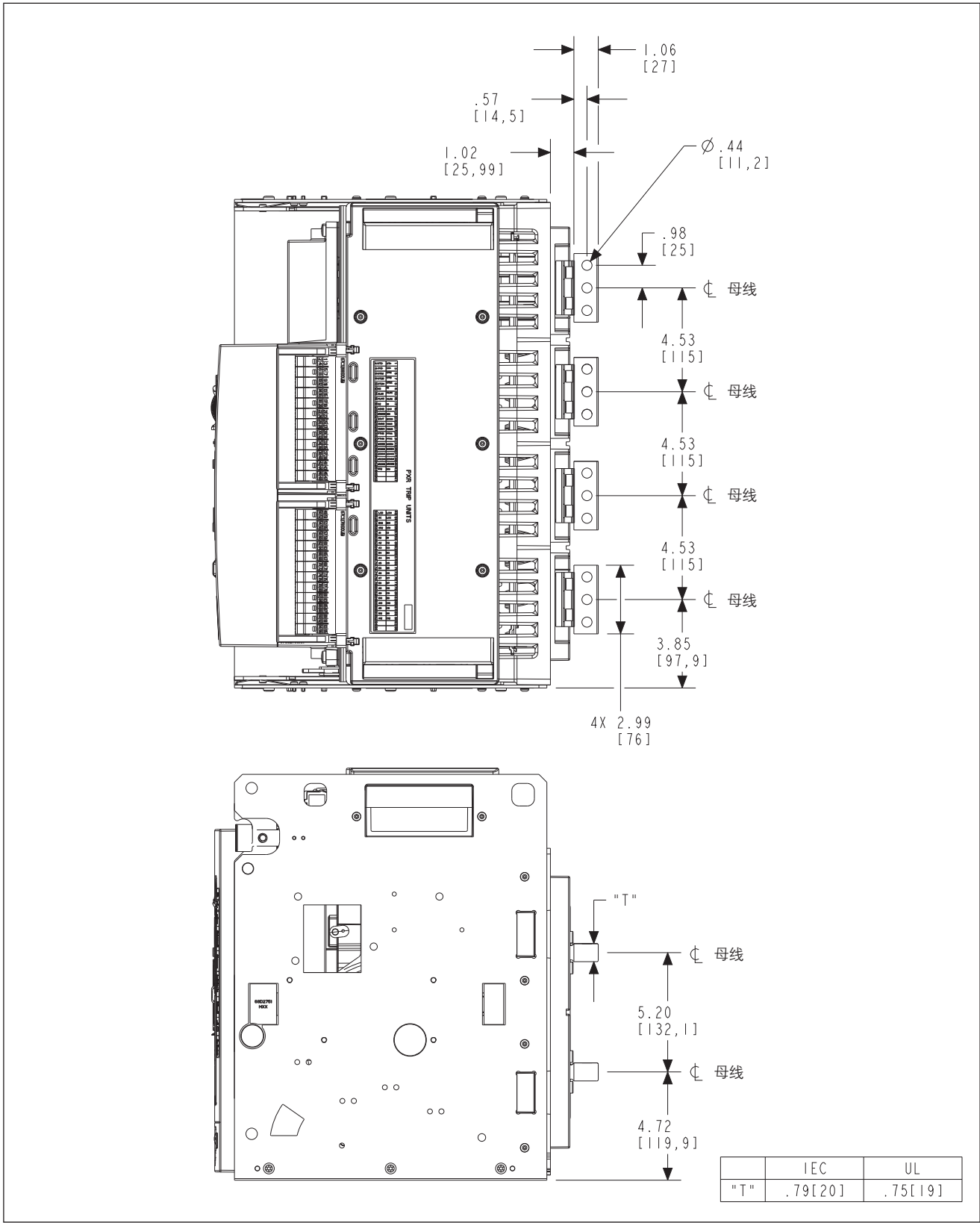
图43. 4极抽出式抽屉座 - 顶视图/侧视图、居中式3孔水平母线适配器。单位：英寸（毫米）
