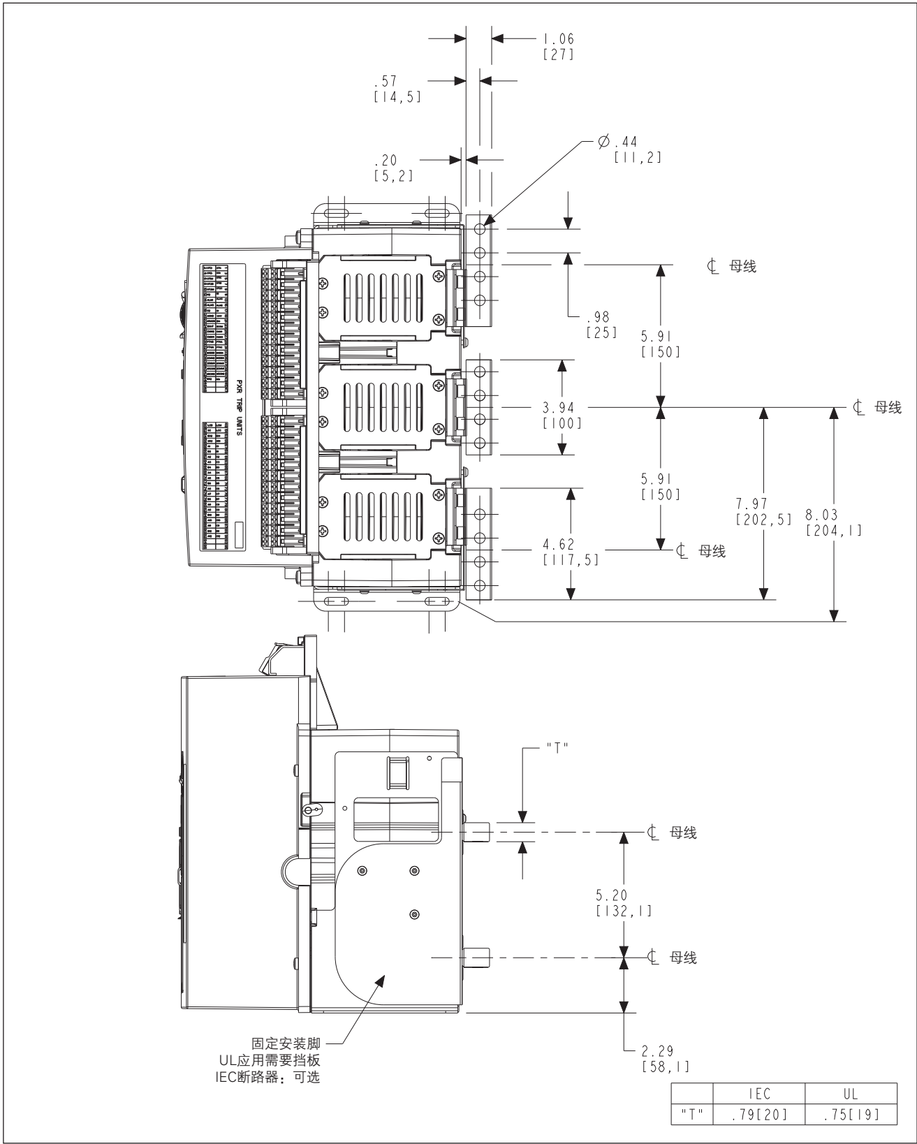
图52. 3极固定式断路- 顶视图/侧视图、偏置4孔水平母线适配器、单位：英寸（毫米）
