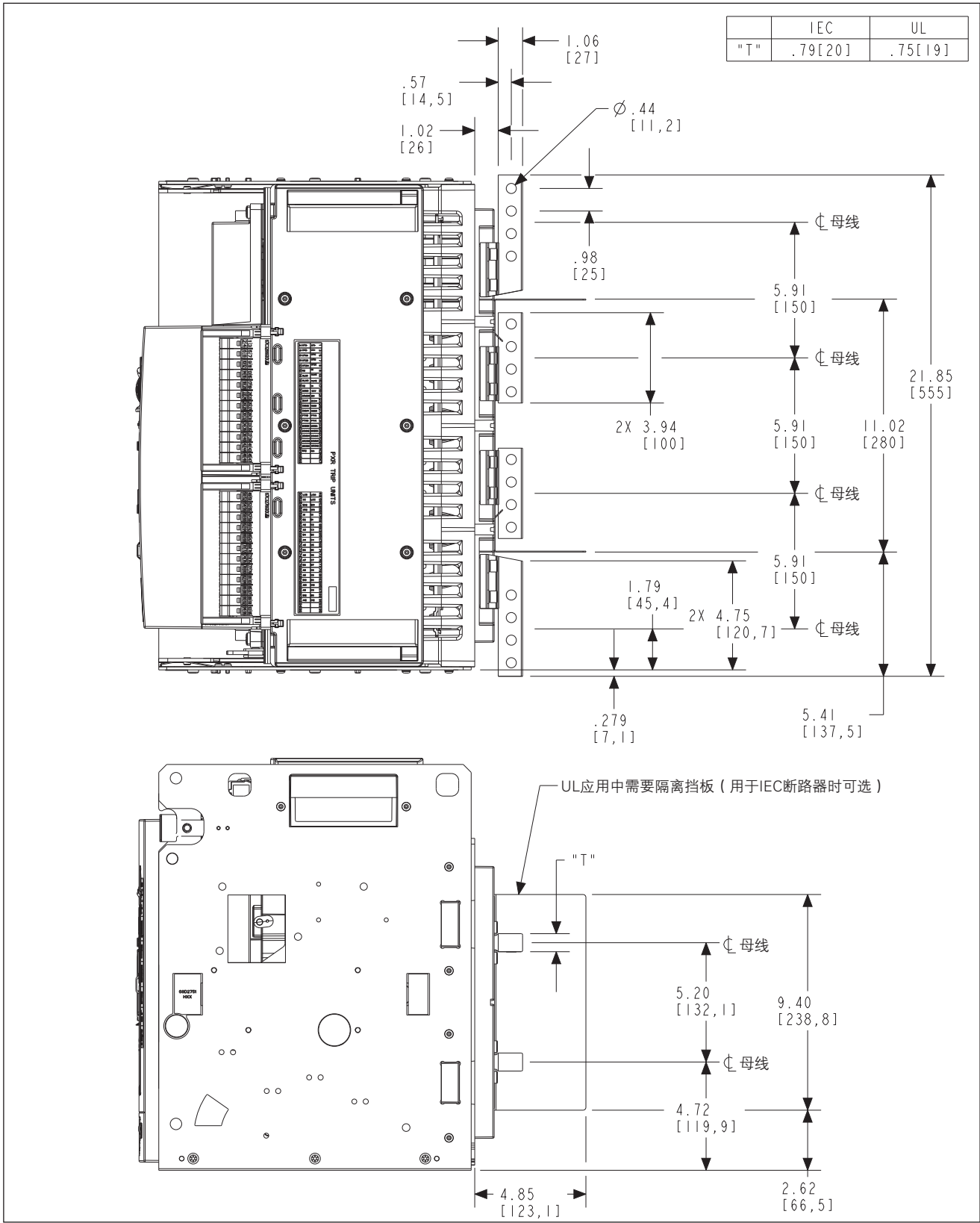
图45. 4极抽出式抽屉座- 顶视图/侧视图、偏置4孔水平母线适配器。单位：英寸（毫米）
