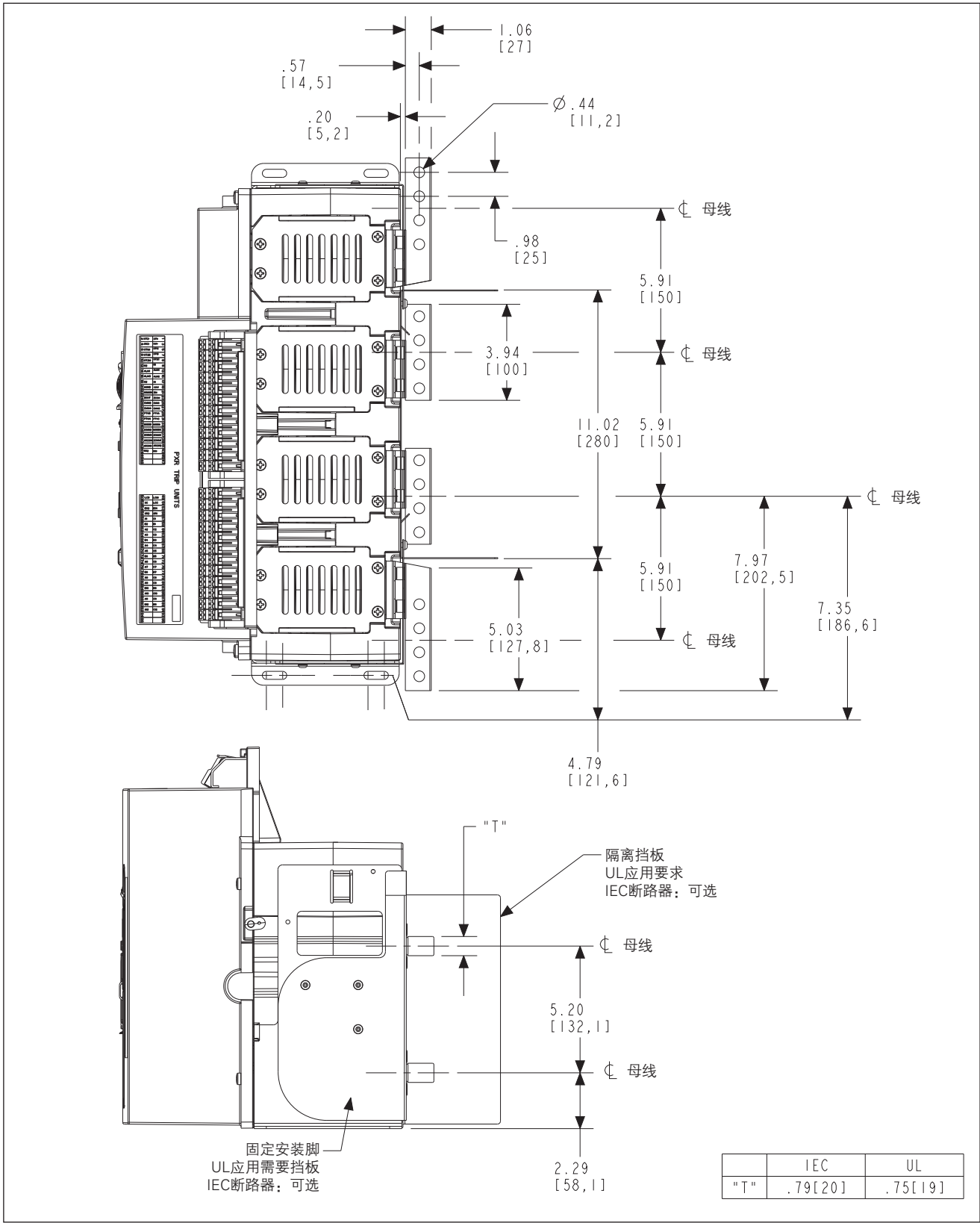
图58. 4极固定式断路器 – 顶视图/侧视图、偏置4孔水平母线适配器、单位：英寸（毫米）
