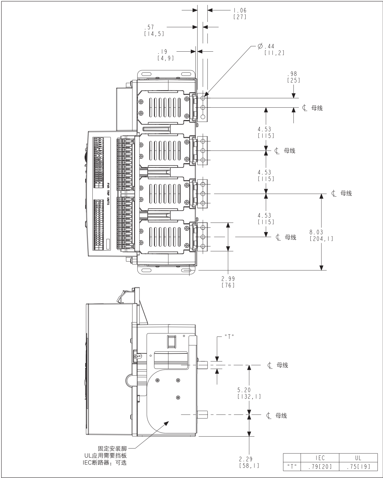
图56. 4极固定式断路器 – 顶视图/侧视图、居中式3孔水平母线适配器。单位：英寸（毫米）
