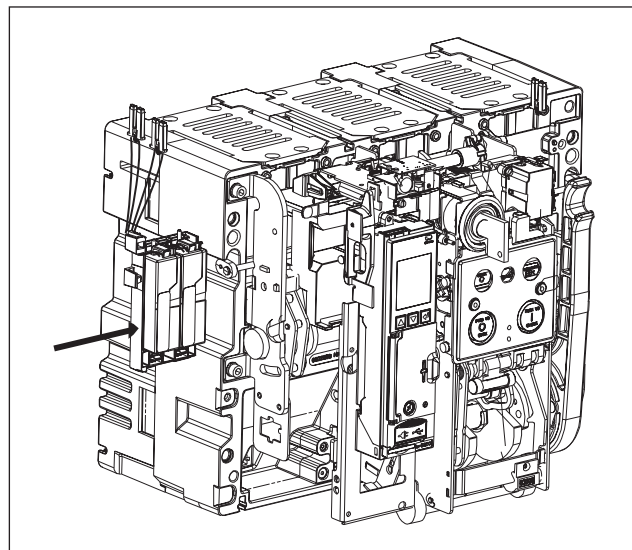
图32. 右侧附件盘
