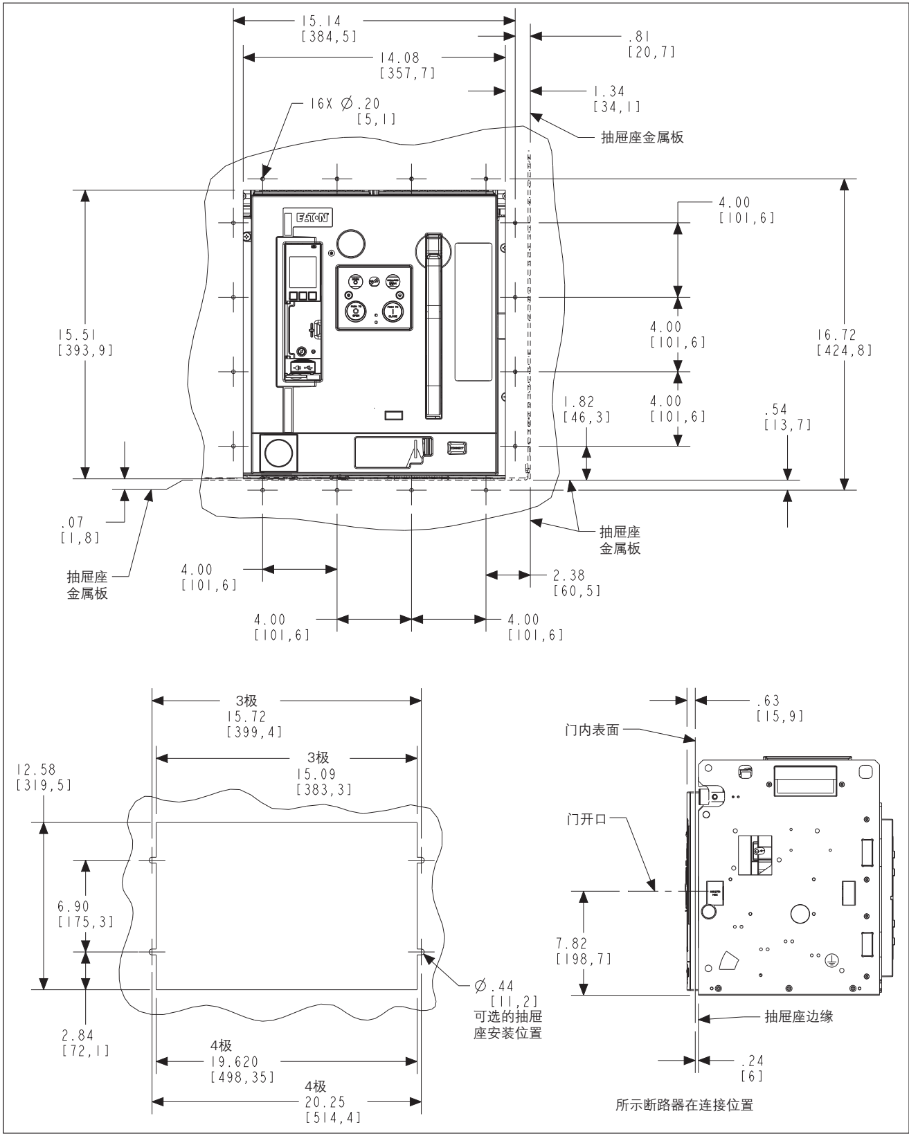
图47. 3极/4极抽出式抽屉座 - 前门开口信息。单位：英寸（毫米）
