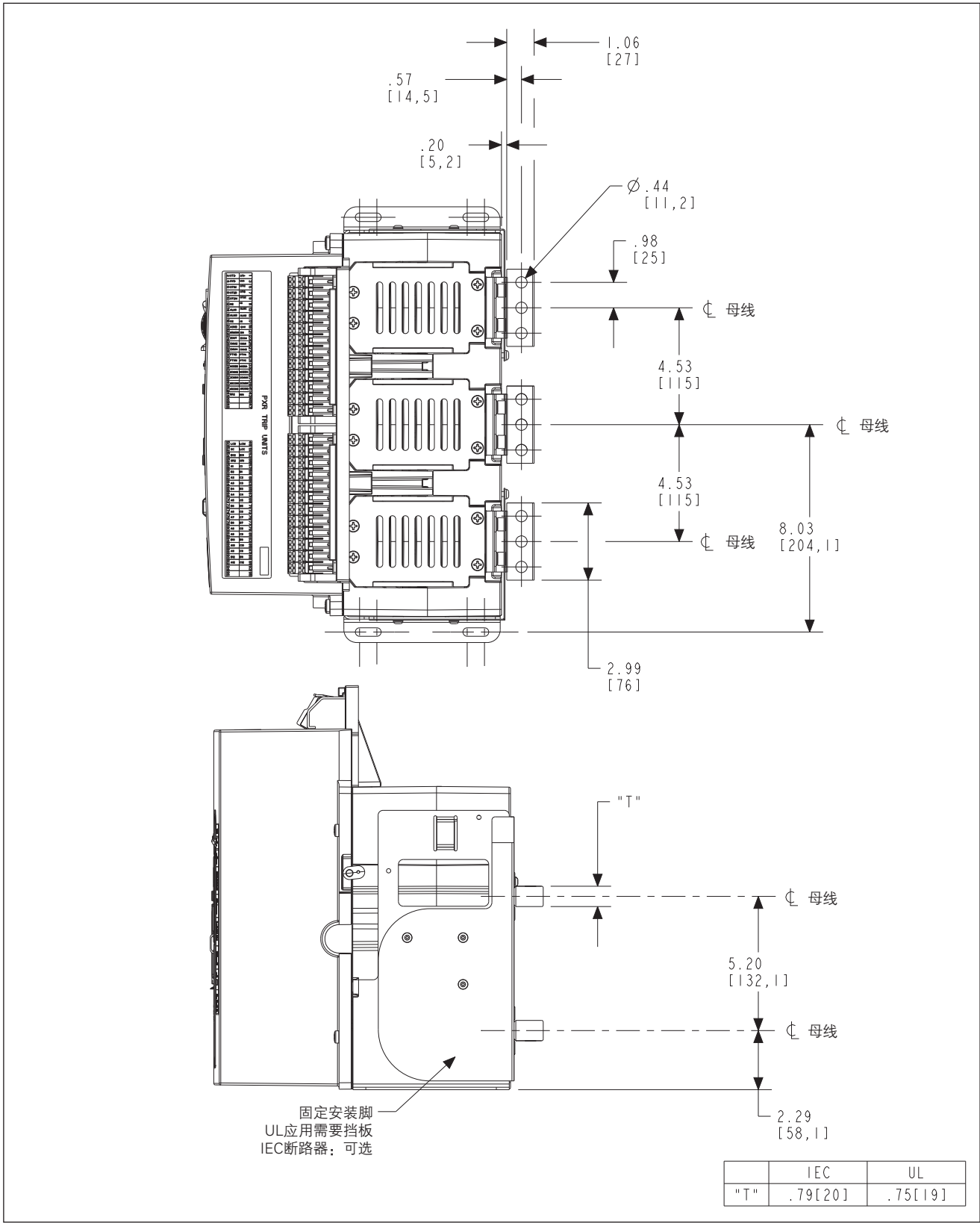
图50. 3极固定式断路器 - 顶视图/侧视图、居中式3孔水平母线适配器。单位：英寸（毫米）
