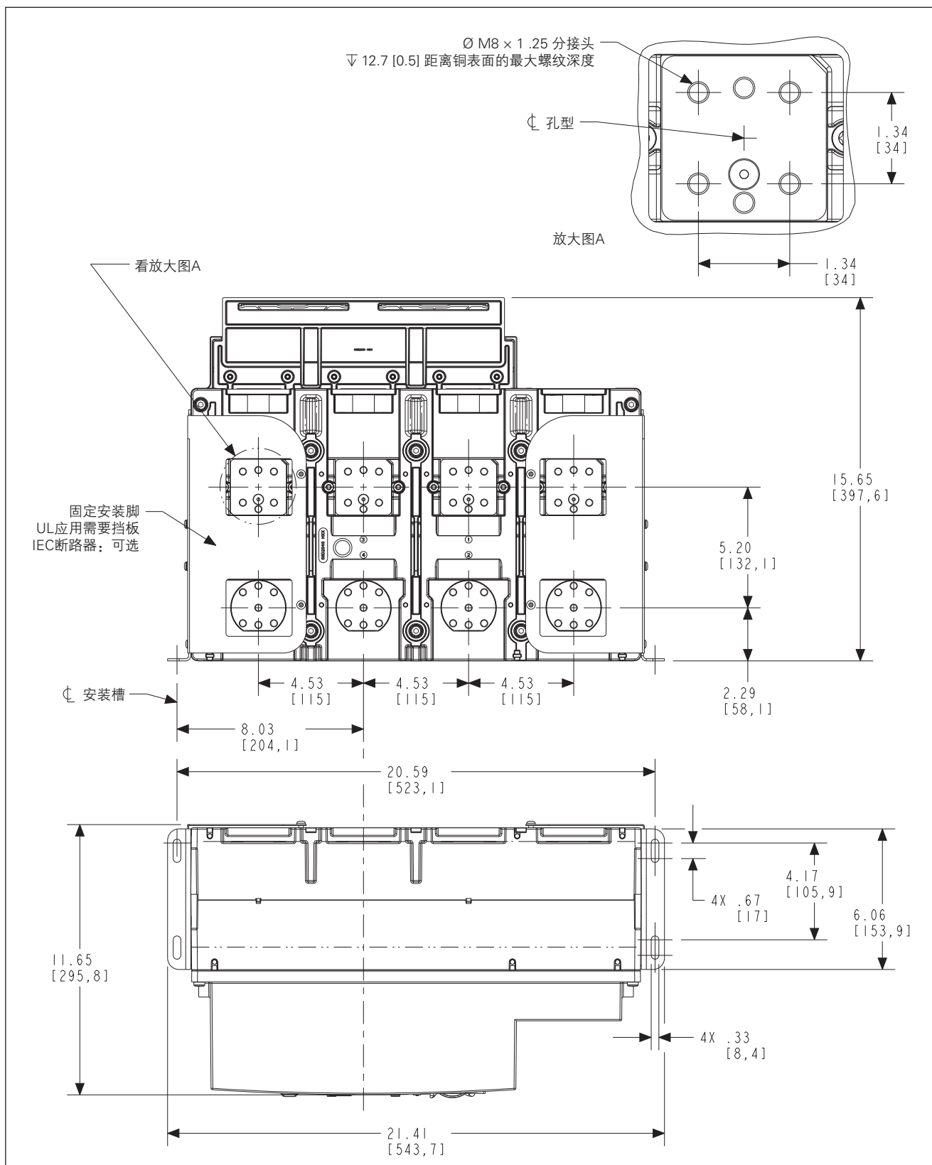
图54. 4极固定式断路器－后视图/底视图。单位：英寸（毫米）
