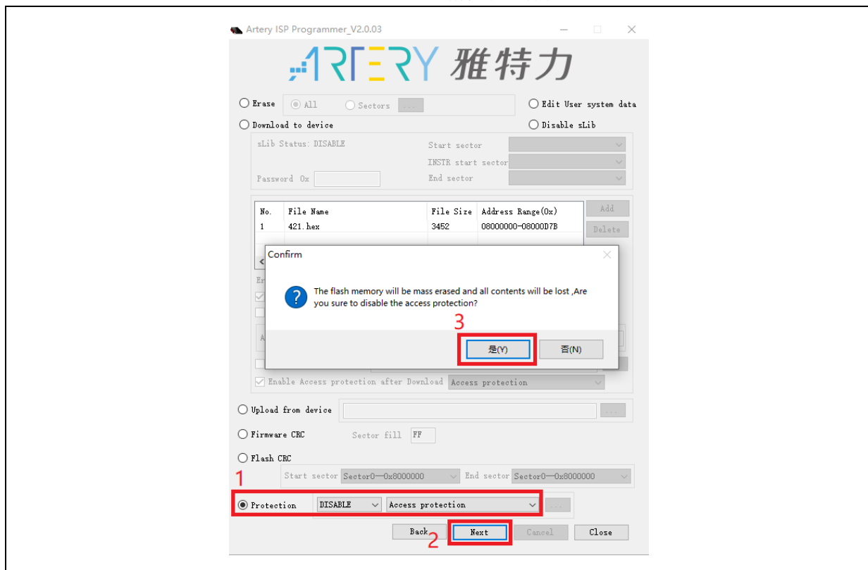
图 23. ISP 工具解除访问保护
