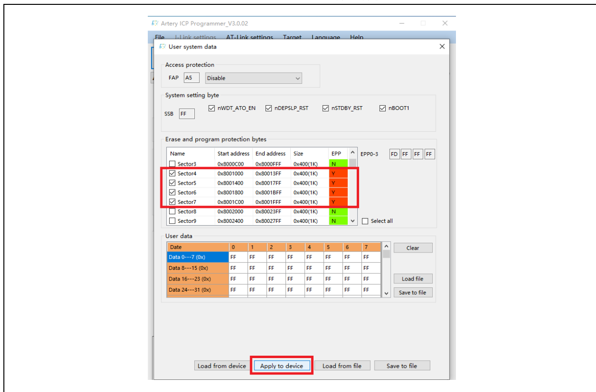
图 24. ICP 工具启用擦写保护
