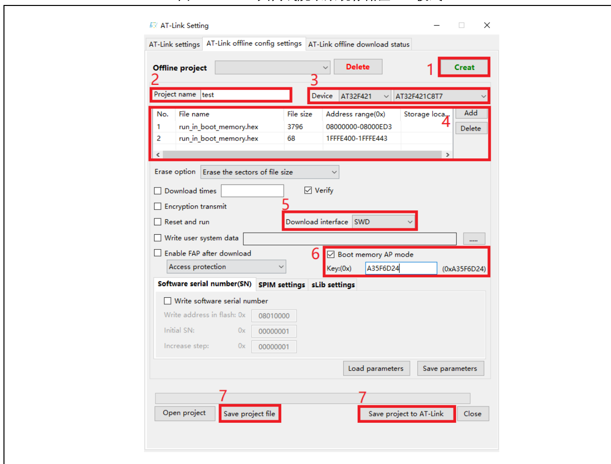
图 28. ICP 工具离线烧录系统存储区 AP 模式
