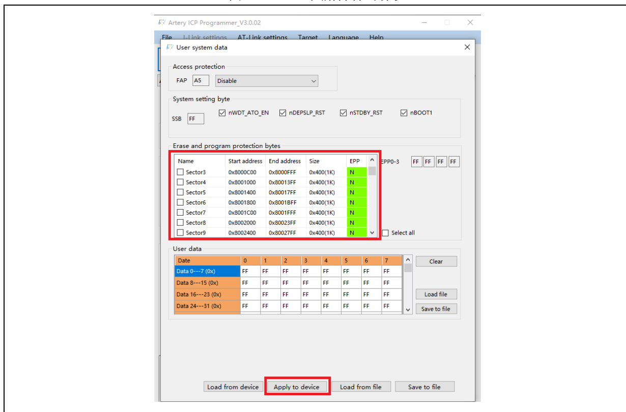
图 25. ICP 工具解除擦写保护
