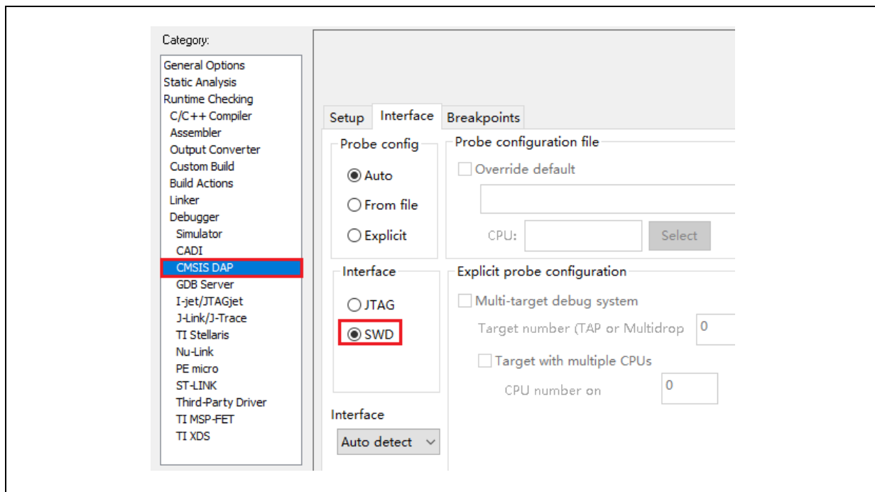
图 15. IAR CMSIS-DAP 选项
