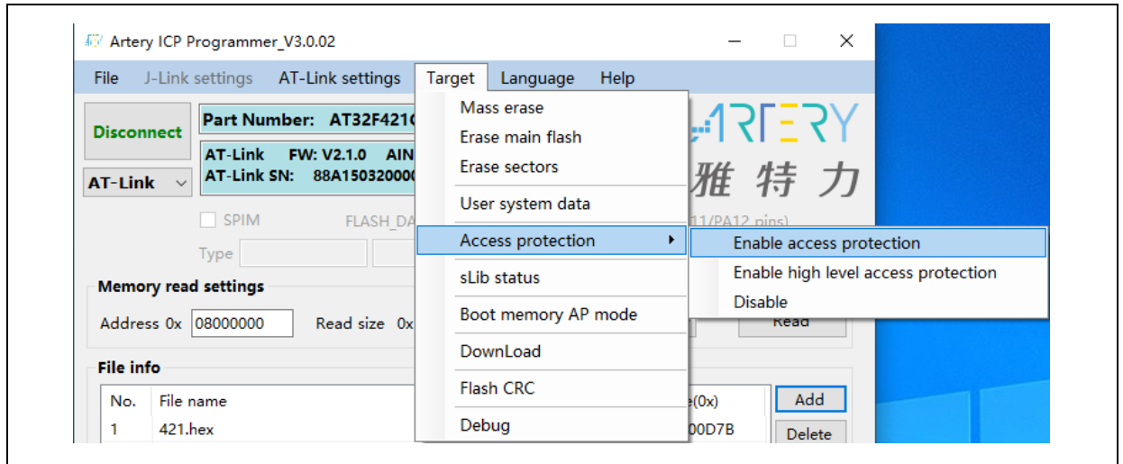
图 21. ICP 工具启用/解除访问保护
