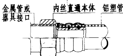
卡(钳)压内丝直通连接
