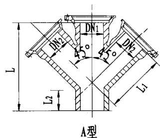
A型Y四通尺寸
