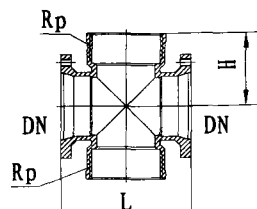
内螺纹四通
