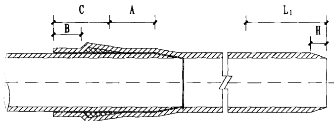
橡胶圈接口
