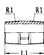
双外螺纹直通
