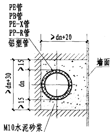
嵌墙安装
