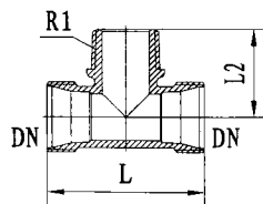
外螺纹三通
