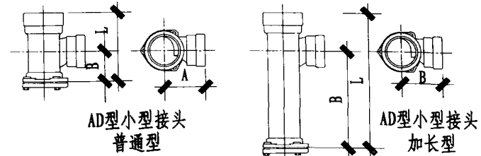
AD型小型接头规格尺寸 (mm)
