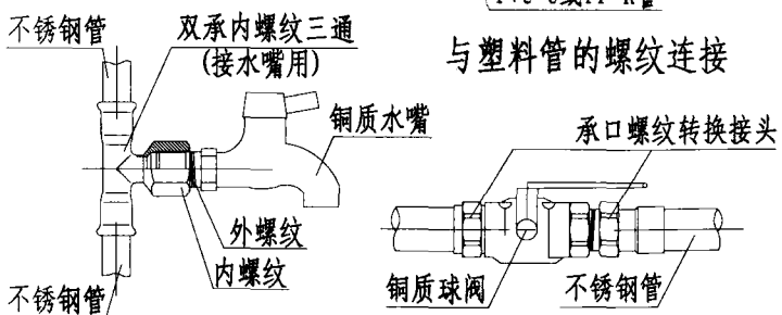
管件与附件连接
