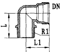
外螺纹90°弯头
