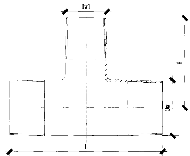
异径三通
