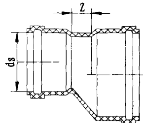
a) 异径
