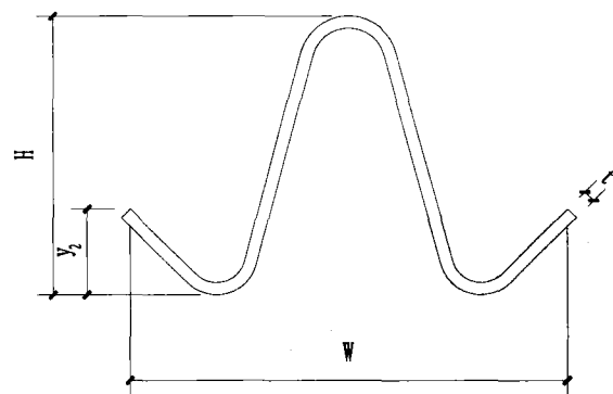
V3型钢筋截面示意图
