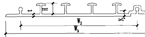
PE板材截面口示意图
