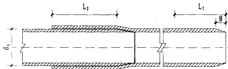
胶粘剂接口
