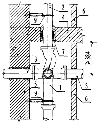
异层安装
