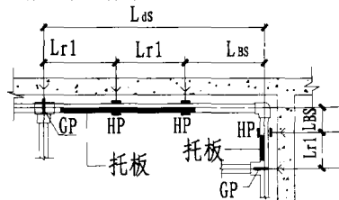
PB管带托板的热水管(热水用)
