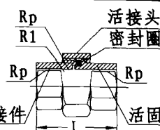
内螺纹活接
