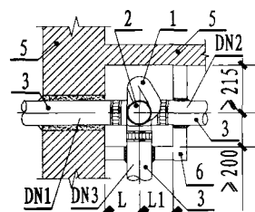
平面安装图
