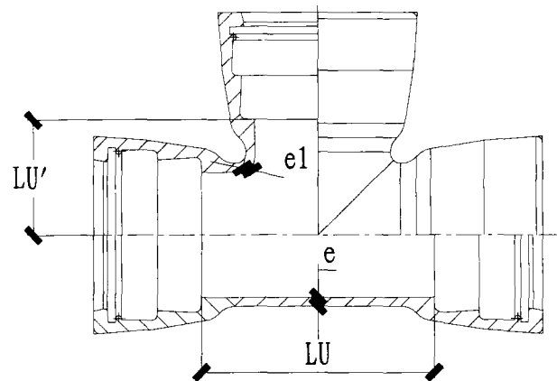
全承三通管件
