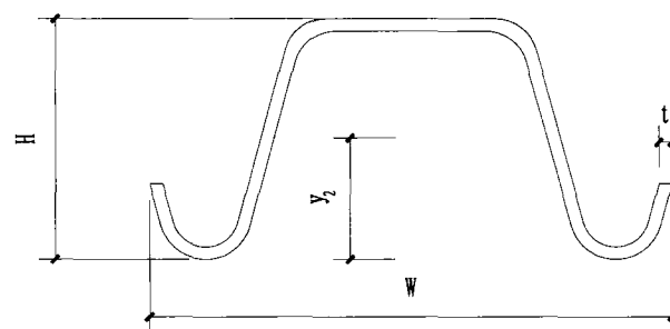
V4型钢筋截面示意图
