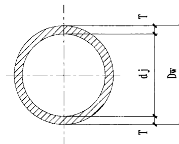
铜管剖面图
