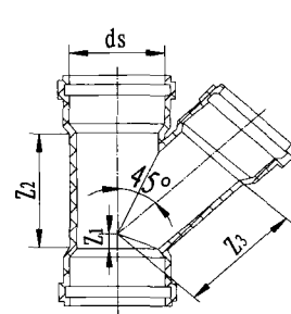
a) 45° 斜三通
