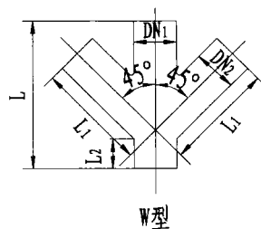
W型Y四通尺寸
