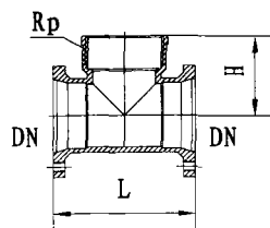
内螺纹三通
