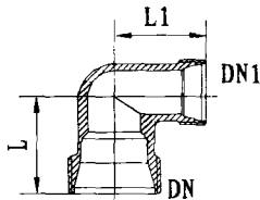
异径90°弯头
