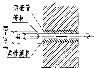
穿内墙
