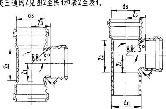
a) 顺水三通
