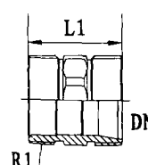
外螺纹直通
