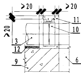
①止水坎节点图
